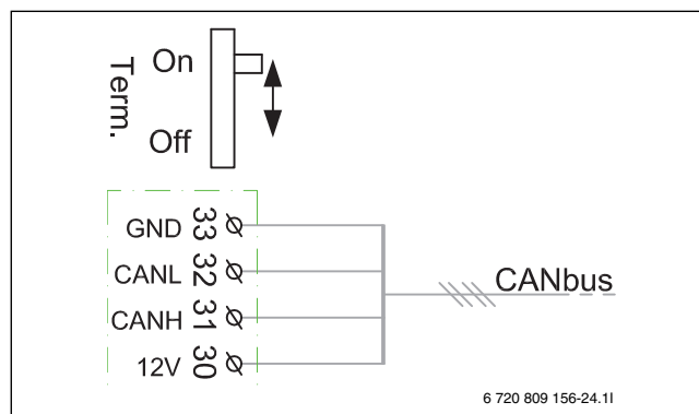
Fig. 7 CAN-BUS-terminering
