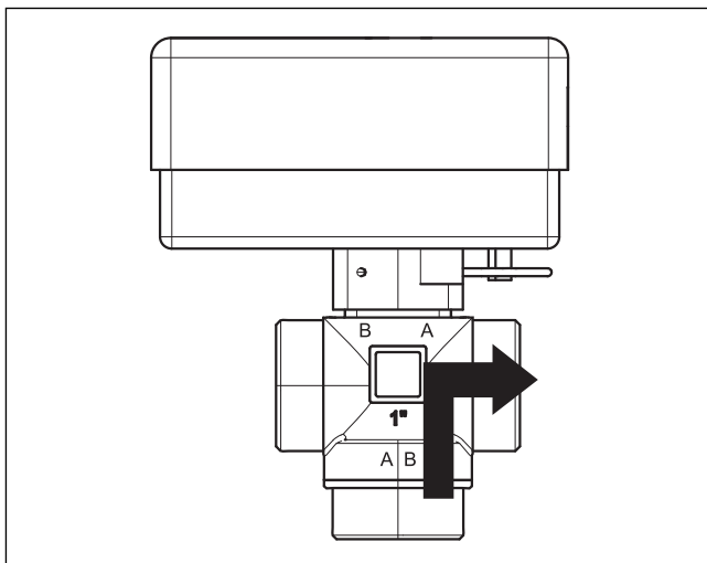
Fig. 21 Lukk kontakt, åpne tilkobling A
