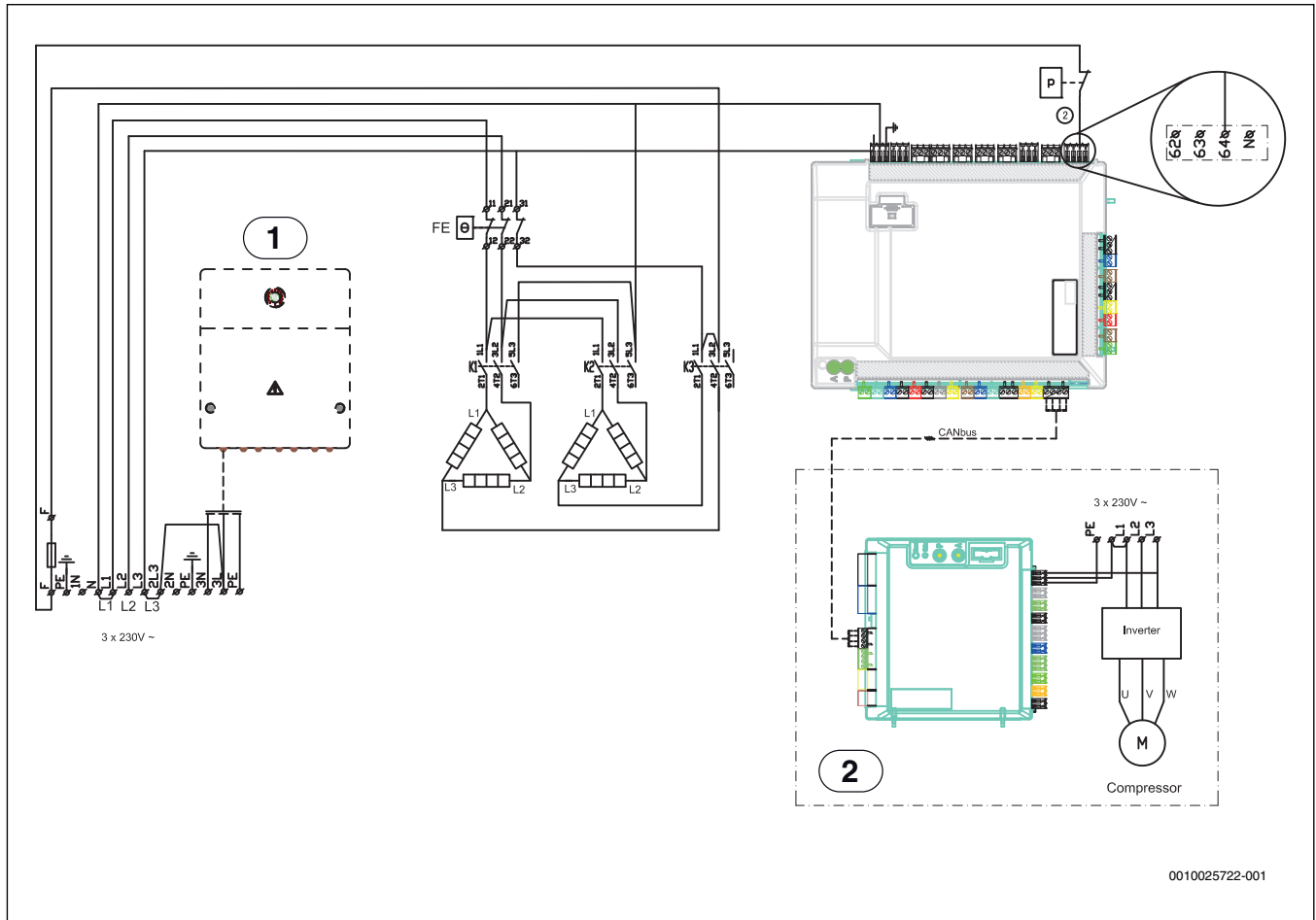
Fig. 12 Koblingsskjema for det elektriske tilskuddet 3 x 230V
