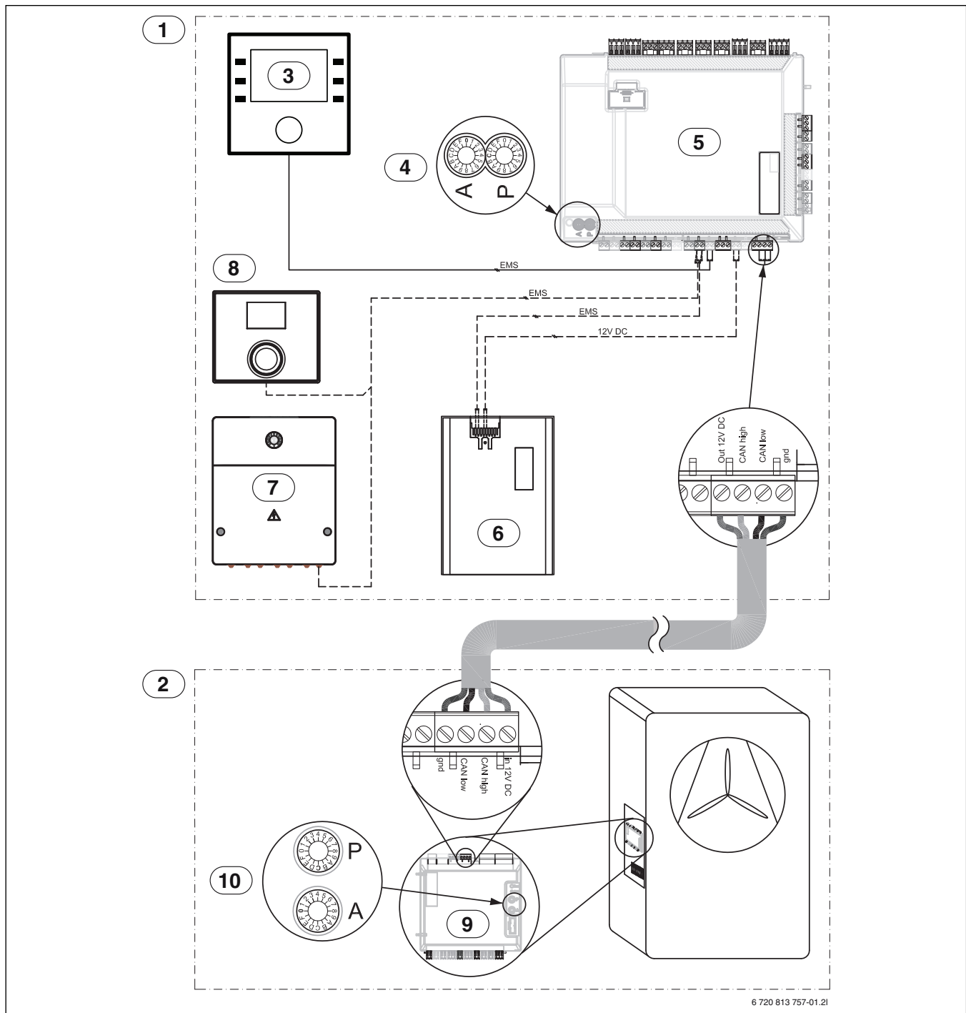
Fig. 29 CAN-BUS/EMS-BUS for innvendig enhet med elektrisk tilskudd – oversikt
