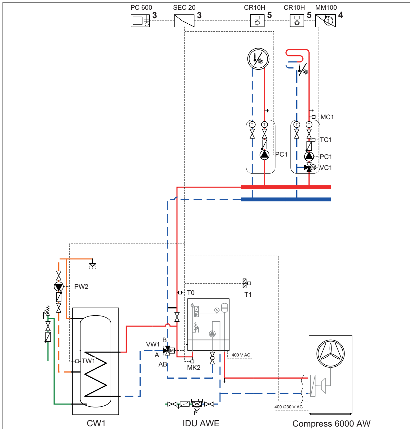
Fig. 28 Elektrisk tilskudd med varmtvannsberederen
