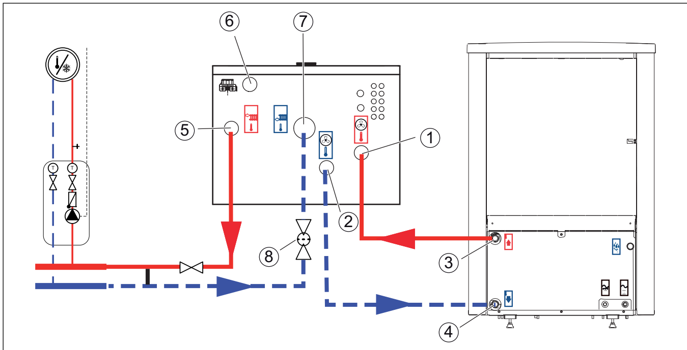
Fig. 5 Tilkobling av den innvendige enheten med elektrisk tilskudd på varmepumpe og varmeanlegg
