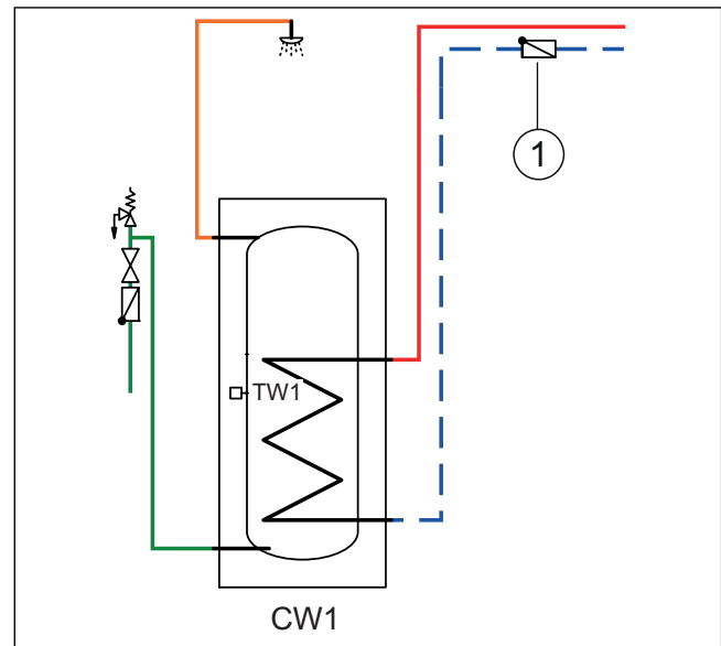
Fig. 19 Varmtvannsbereder
