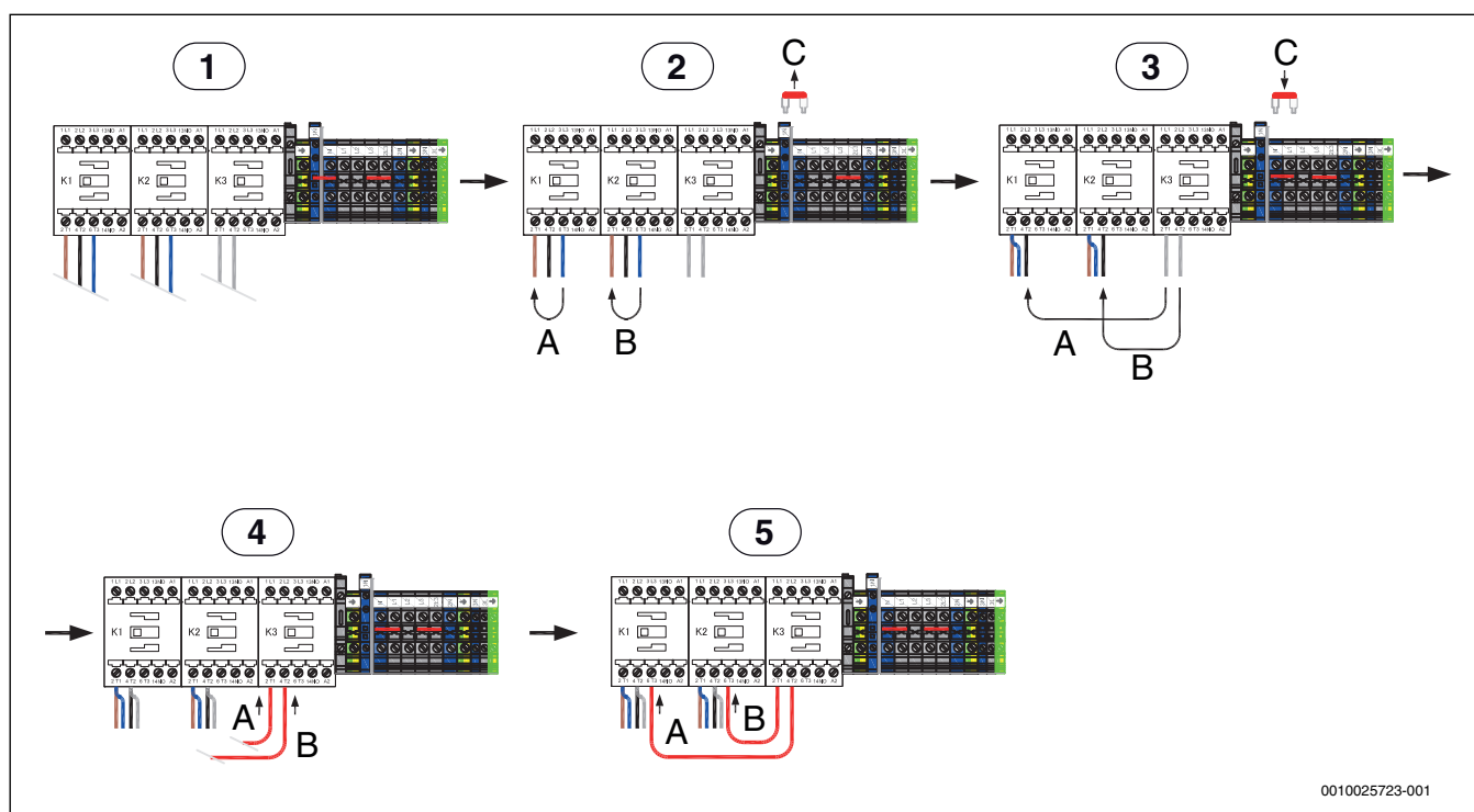
Fig. 13 Omkobling av kontakter i bryterskap
