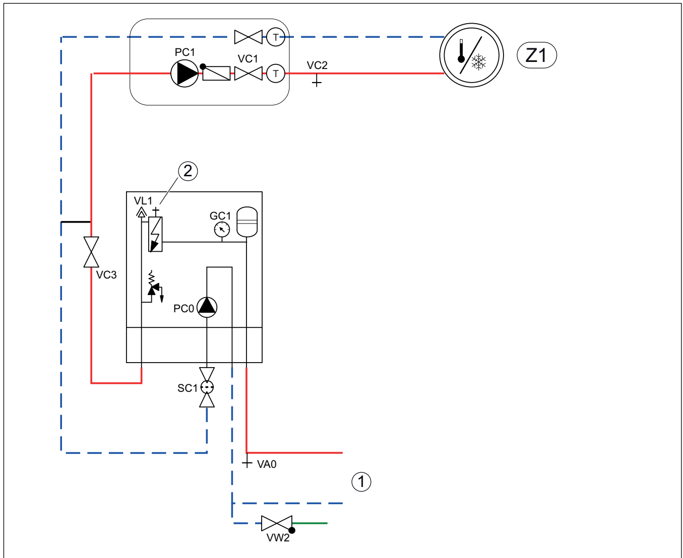
Fig. 16 Innvendig enhet med integrert elektrisk tilskudd og varmesystem
