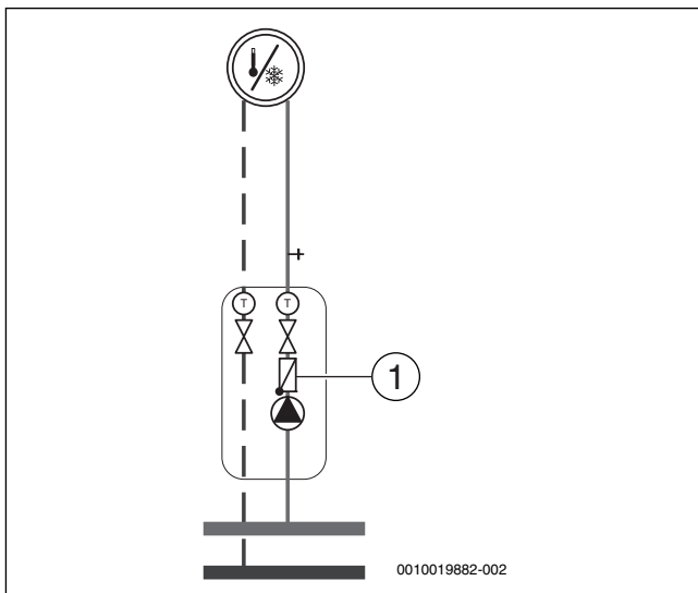
Fig. 27 Varmekrets
