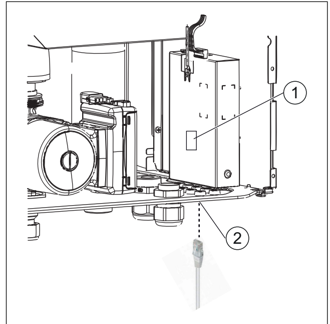
Fig. 25 IP-modul
