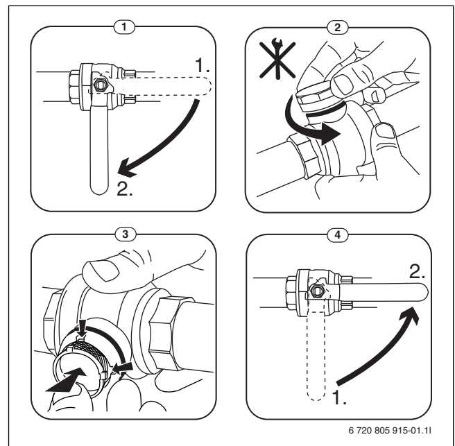
Fig. 17 Rengjøring av sil
