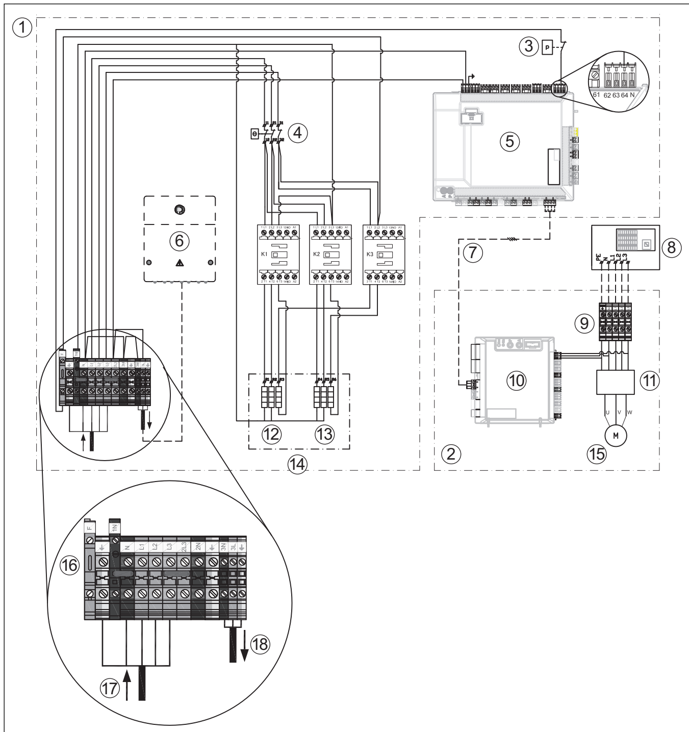
Fig. 31 Varmepumpe (trefase vekselstrøm) med integrert elektrisk tilskudd (trefase vekselstrøm)
