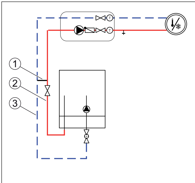
Fig. 26 Innvendig enhet med varmekrets og bypass
