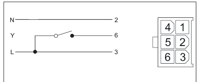
Fig. 23 Molex-støpsel
