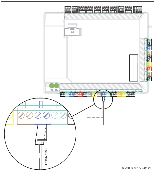
Fig. 18 EMS-tilkobling på installasjonsmodulen
