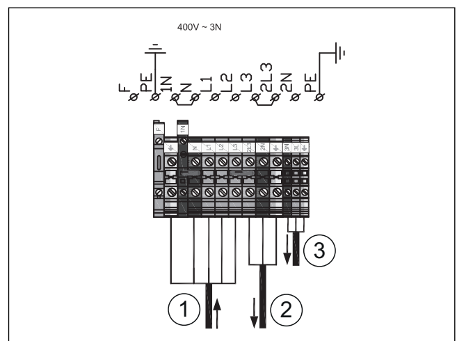
Fig. 10 Elektrisk standardtilkobling ved integrert elektrisk tilskudd
