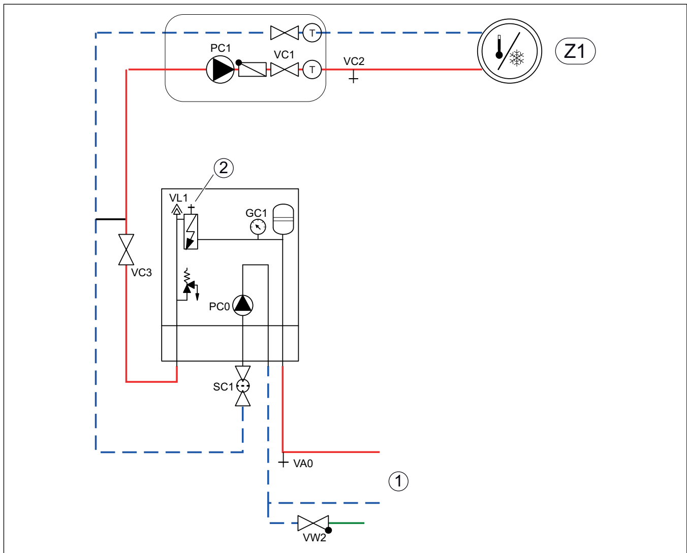
Fig. 6 Innvendig enhet med integrert elektrisk tilskudd og varmesystem
