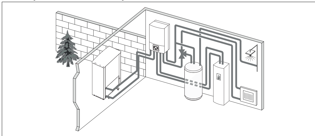
Fig. 3 Varmepumpe Compress 6000 AW innvendig enhet AWB uten elektrisk tilskudd, ekstern varmtvannsbereder og eksternt tilskudd
