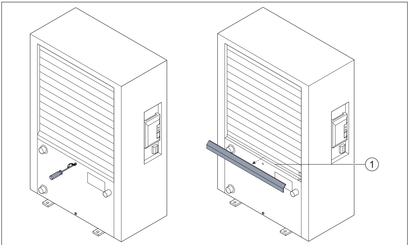
Fig. 8 Varmepumpens kondensbeholder
