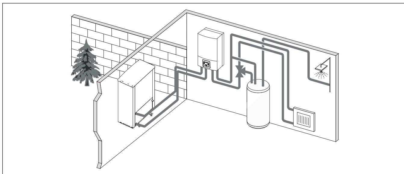
Fig. 3 Varmepumpe Compress 6000 AW med innvendig enhet AWE med elektrisk tilskudd og ekstern varmtvannsbereder
