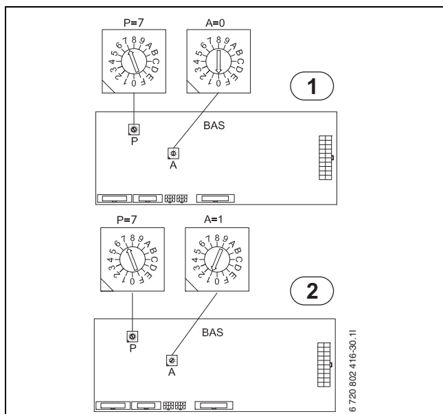
Fig. 73 Adressering av varmepumpe 1 og 2
