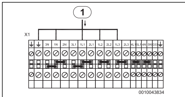
Fig. 64 Standard design C6–C11 og E6–E11
