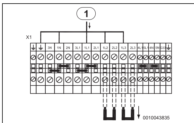
Fig. 65 Elektrisk tilskudd 1 kW, C6–C11 og E6–E11
