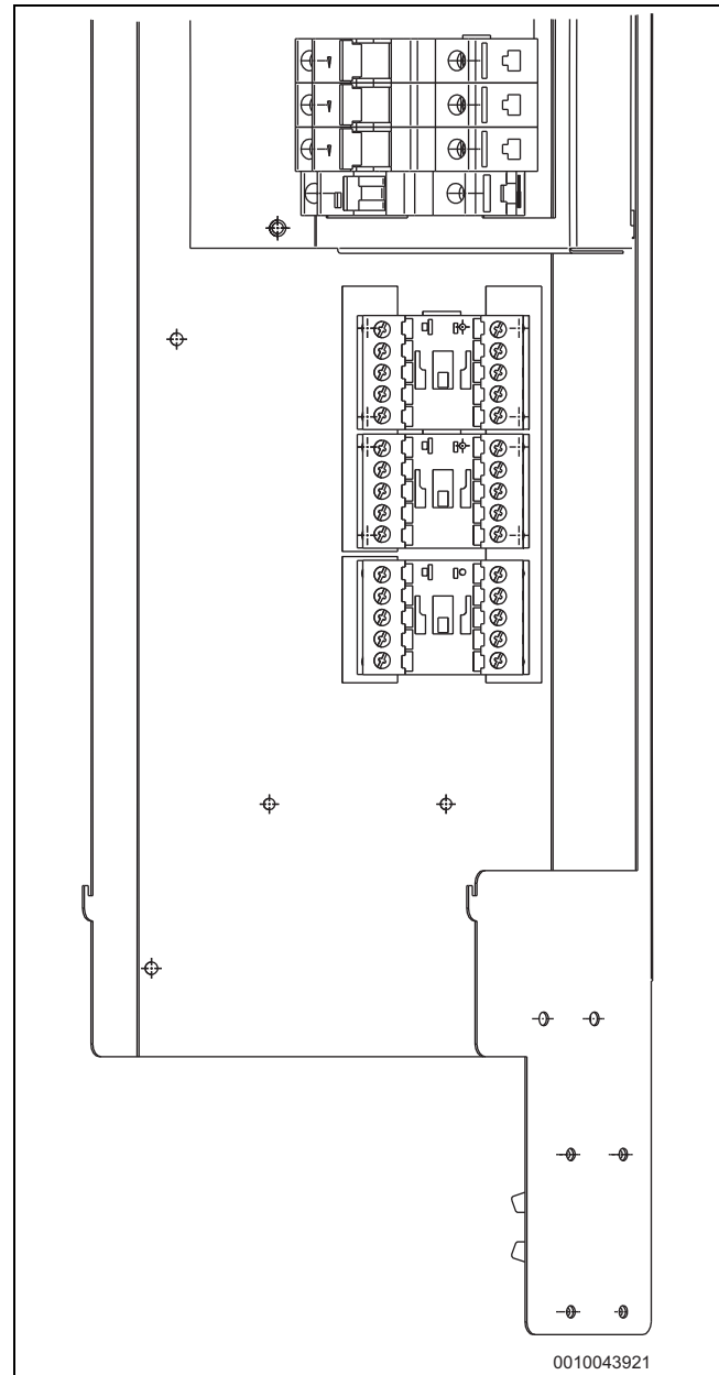
Fig. 41 Opphengsskinne
