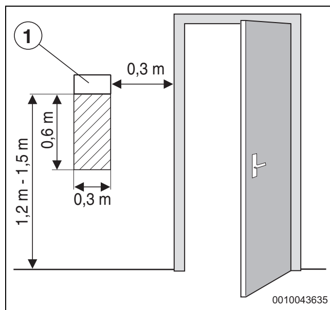
Fig. 39 Anbefalt plassering av romtemperaturføler
