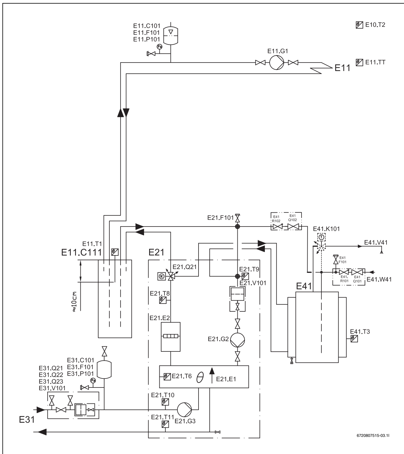
Fig. 56 Ushuttet varmekrets med akkumulatortank og ekstern varmtvannsbereder
