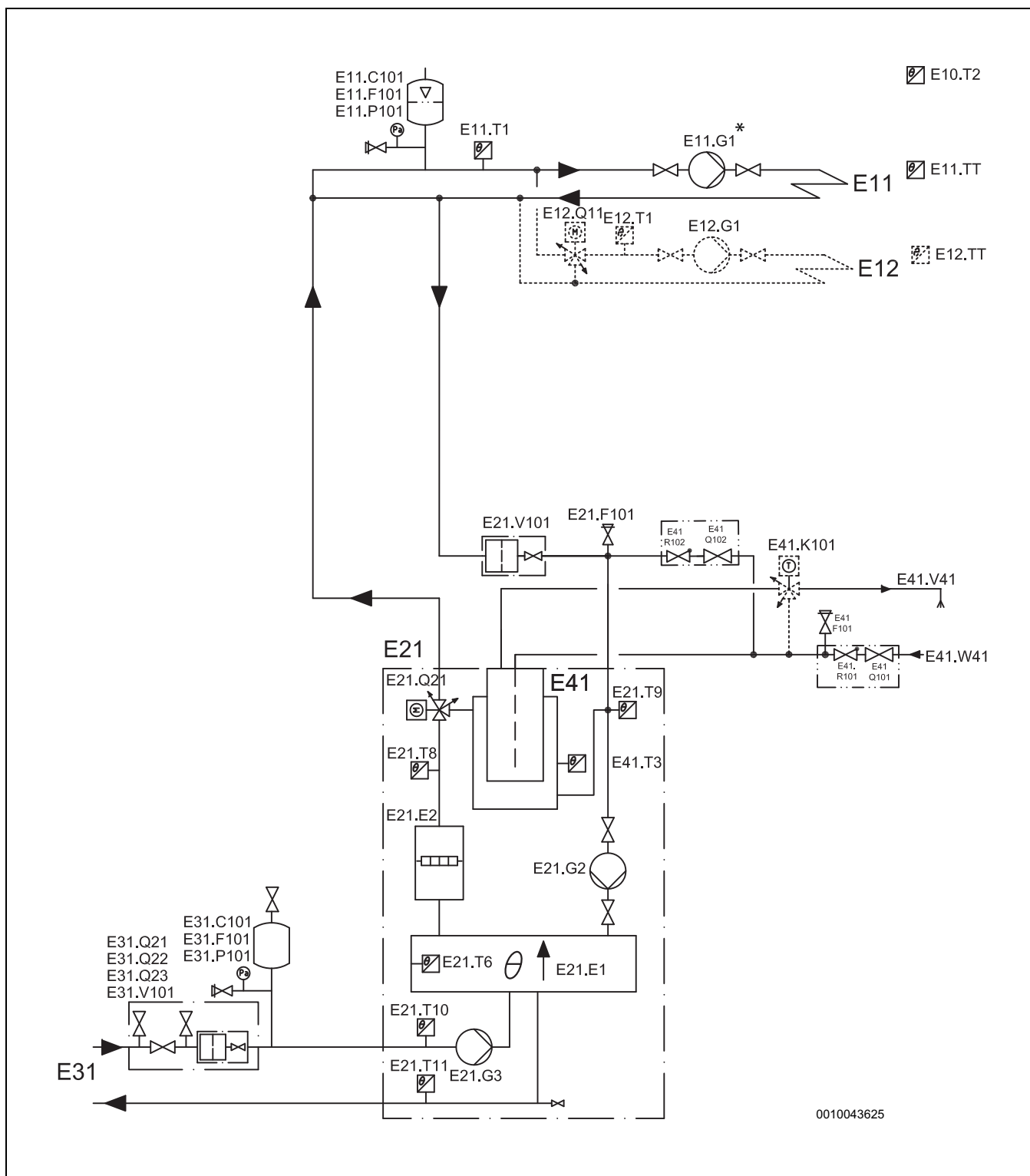
Fig. 55 Varmekrets uten og med shunt
