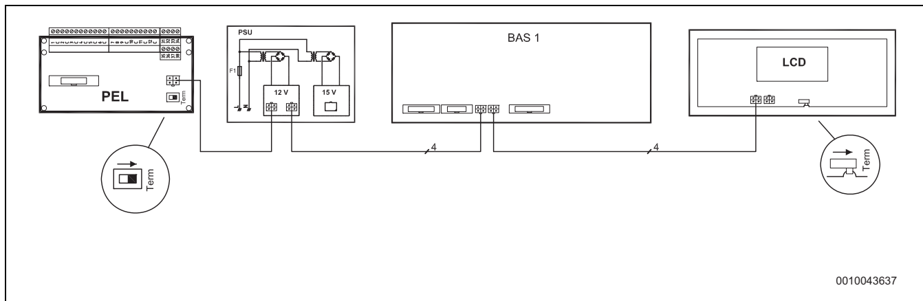
Fig. 59 CAN-busoversikt
