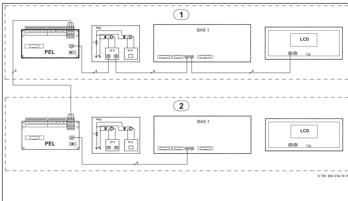
Fig. 72 CAN-busoversikt med to varmepumper
