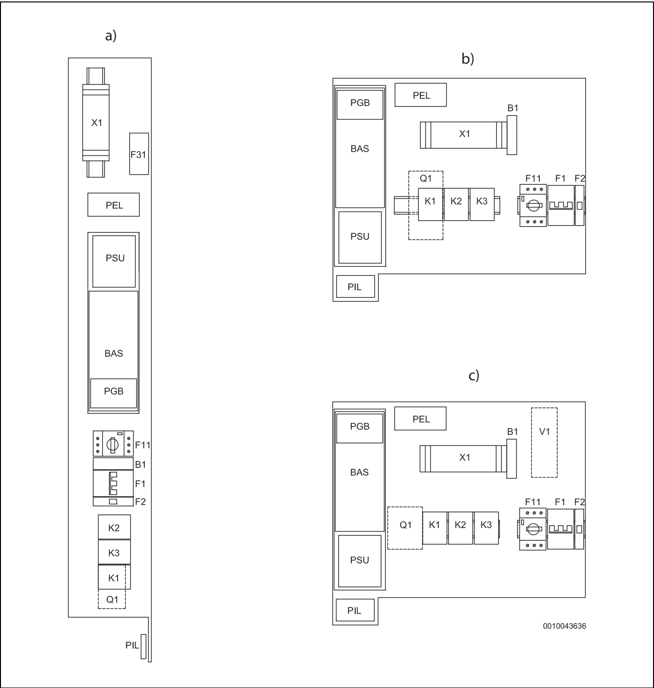
Fig. 58 Oversikt, kretskort
