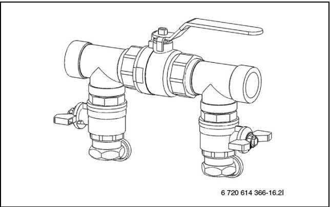
Fig. 16 Påfyllingsanordning 14-17 LW
