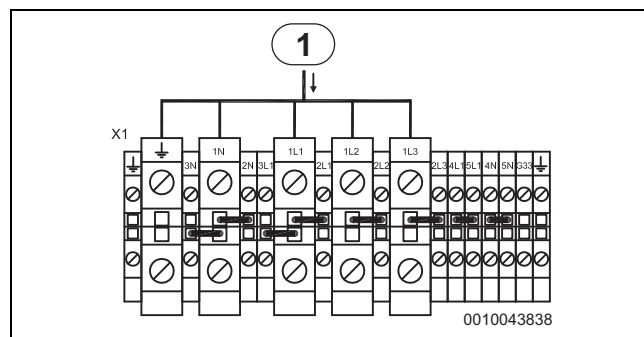
Fig. 68 Standard design E14–E17
