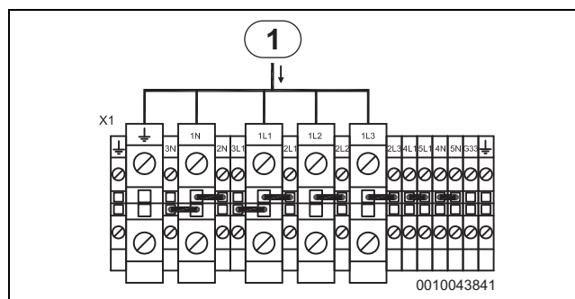
Fig. 71 Elektrisk tilskudd 3 kW, E14–E17
