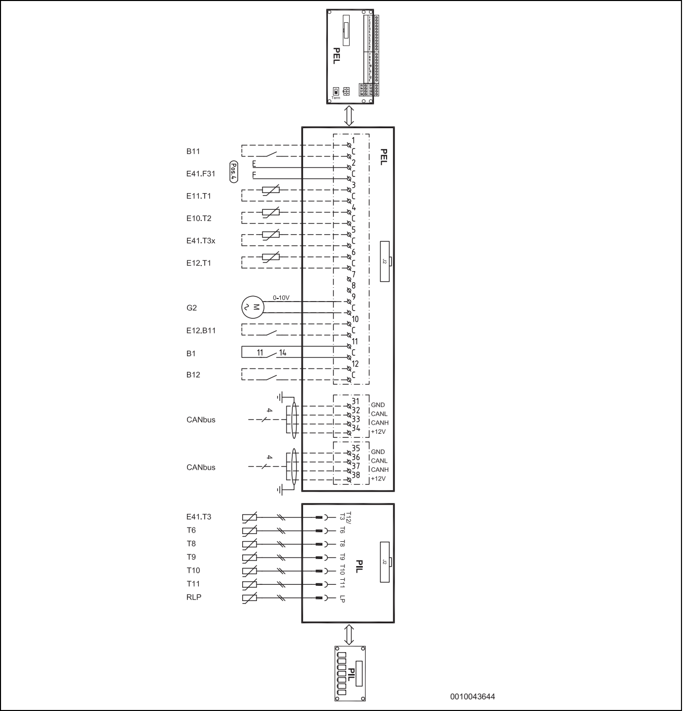
Fig. 63 Komplette tilkoblingsskjemakoblinger (230 V)
