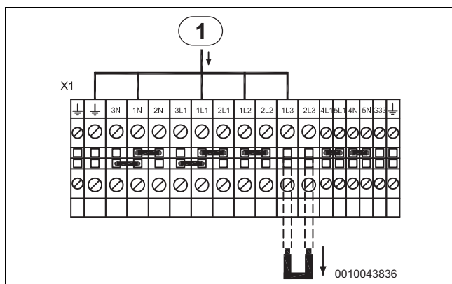
Fig. 66 Elektrisk tilskudd 2 kW, C6–C11 og E6–E11
