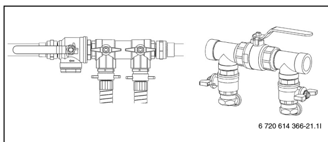
Fig. 22 Påløpingsanordninger i normal posisjon
