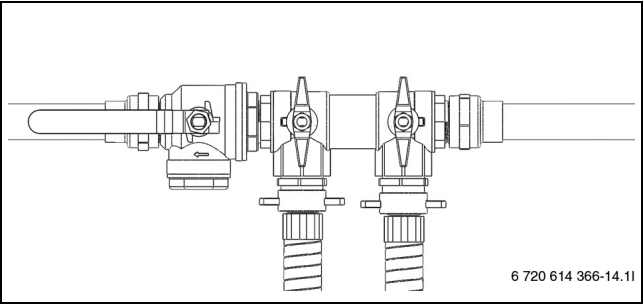
Fig. 15 Påfyllingsanordning 6-11 LWM, 6-17 LW
