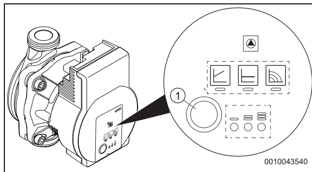
Fig. 7 Kuldebærerpumpe (Para)
