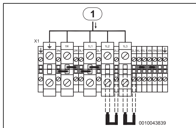
Fig. 69 Elektrisk tilskudd 1 kW, E14–E17
