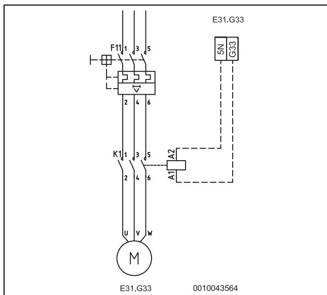
Fig. 14 Tilkobling, grunnvannspumpe
