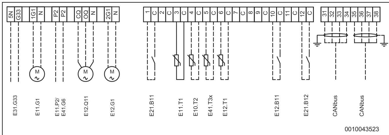
Fig. 13 Eksterne tilkoblinger
