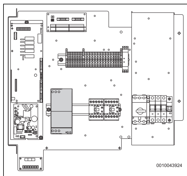
Fig. 44 Startstrømbegrenser installert
