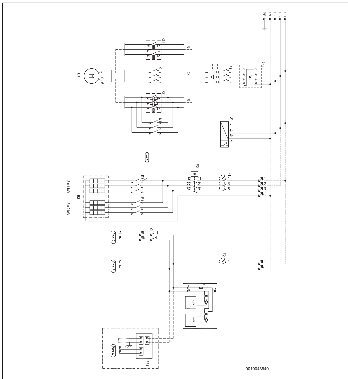
Fig. 61 Internt tilkoblingsskjema
