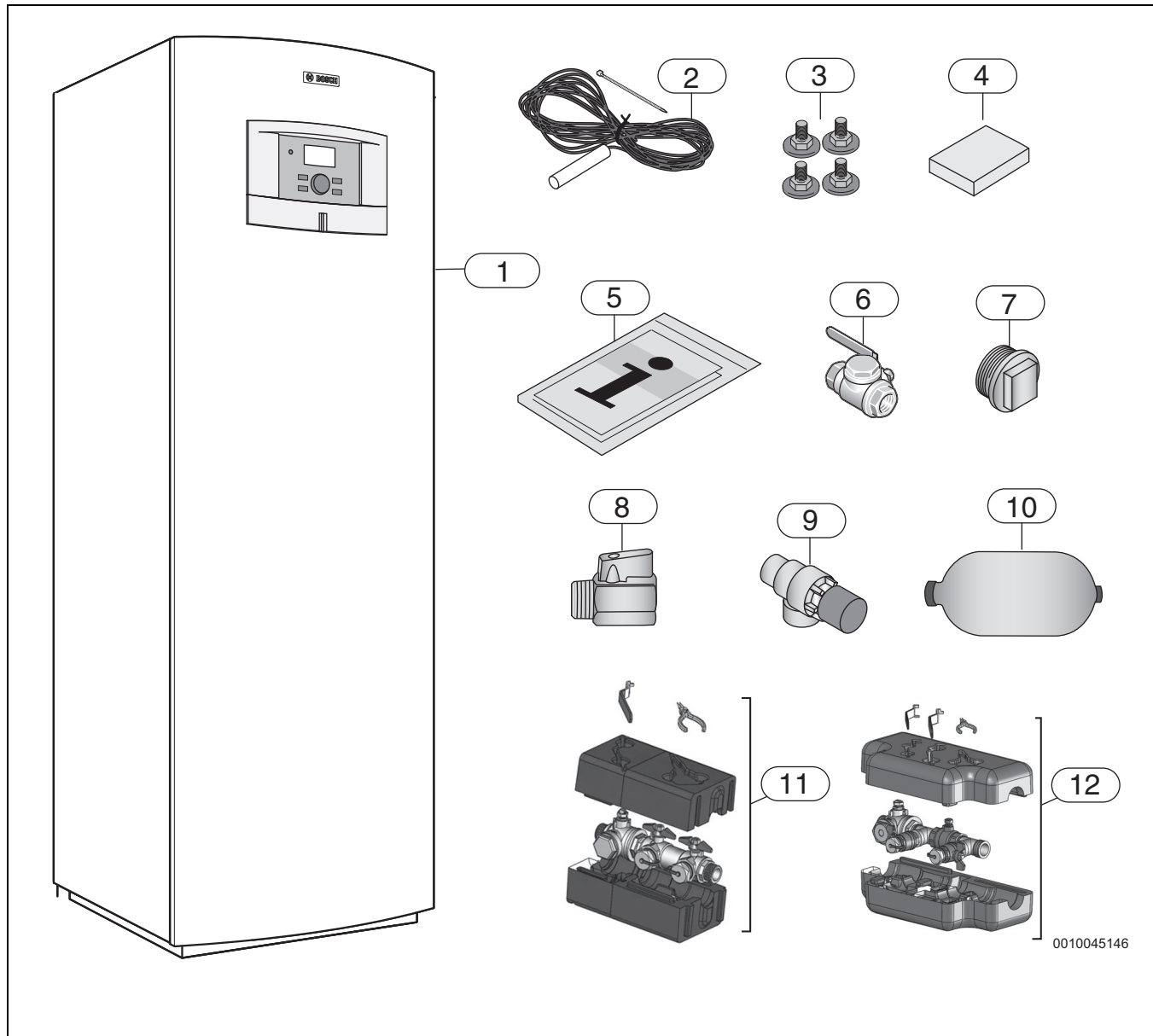
Fig. 2 Medfølgende deler
