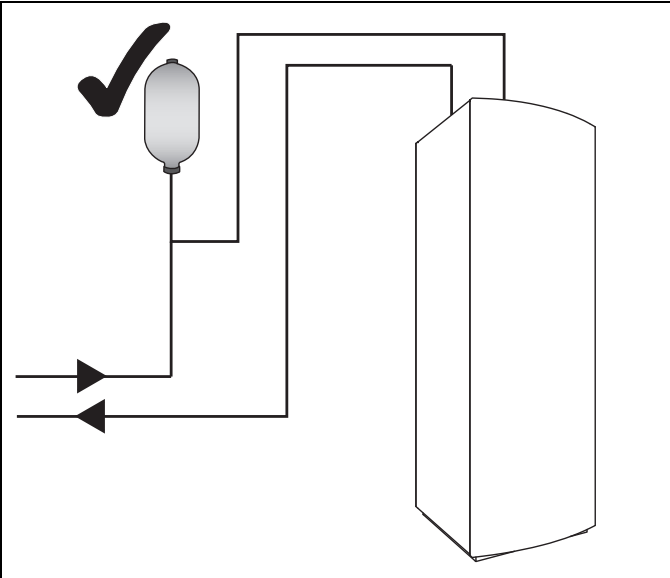
Fig. 10 Montering av et ekspansjonskar
