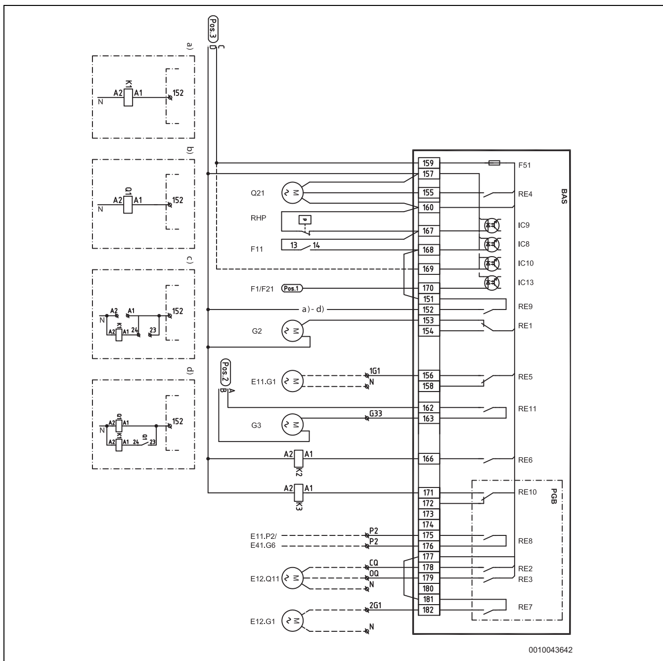
Fig. 62 Komplette tilkoblingsskjemakoblinger (230 V)
