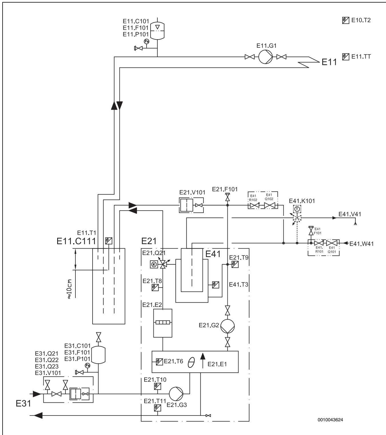
Fig. 54 Ushuntet varmekrets uten akkumulatortank
