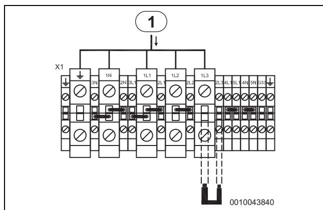
Fig. 70 Elektrisk tilskudd 2 kW, E14–E17
