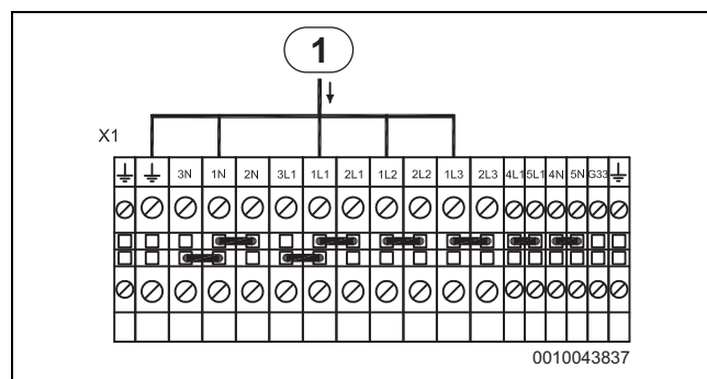
Fig. 67 Elektrisk tilskudd 3 kW, C6–C11 og E6–E11
