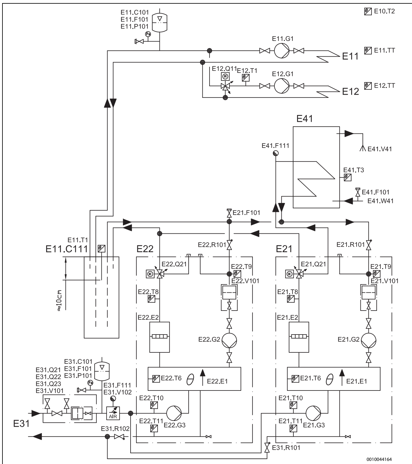
Fig. 57 To varmepumper (seriekobling) med varmekrets med og uten shunt, akkumulatortank og ekstern varmtvannsbereder.
