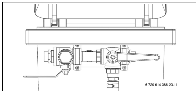
Fig. 20 Påløpingsanordning i fyllerposisjon
