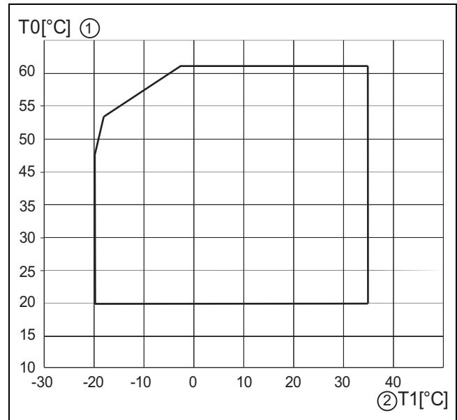
Fig. 1 Varmepumpe uten tilskudd
