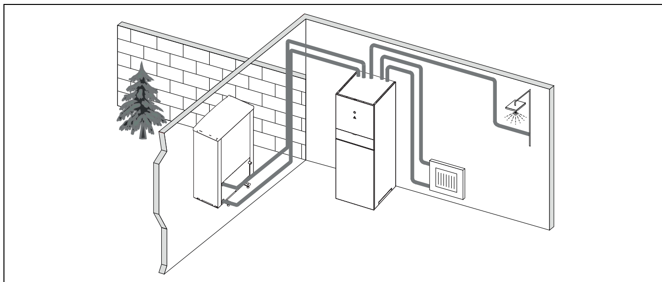
Fig. 3 Varmepumpe Compress 7000i AW, inneenhet AWM / AWMS med integrert varmtvannsbereder og strømtilskudd
