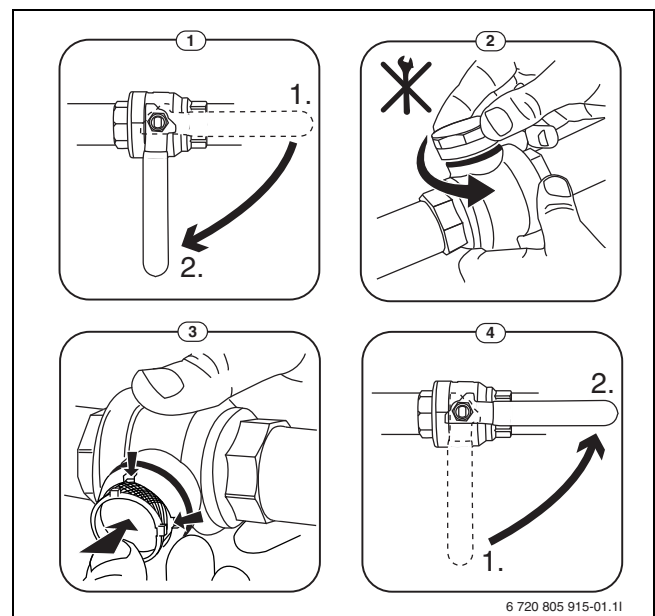
Fig. 8 Rengjøring av sil
