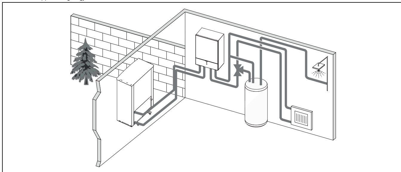
Fig. 3 Varmepumpe Compress 7000i AW, inneenhet AWE med strømtilskudd og ekstern varmtvannsbereder
