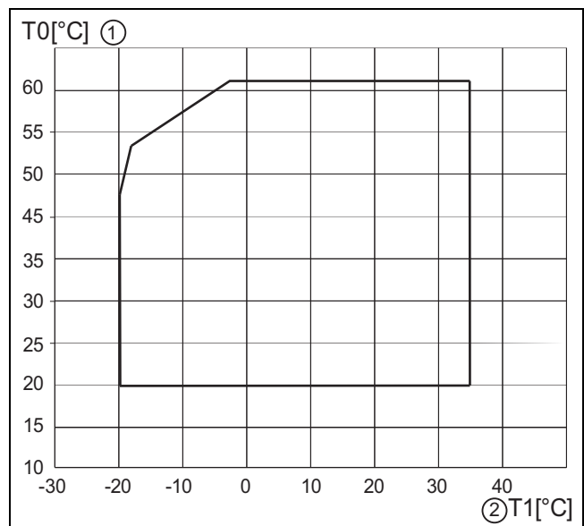
Fig. 1 Varmepumpe uten tilskudd
