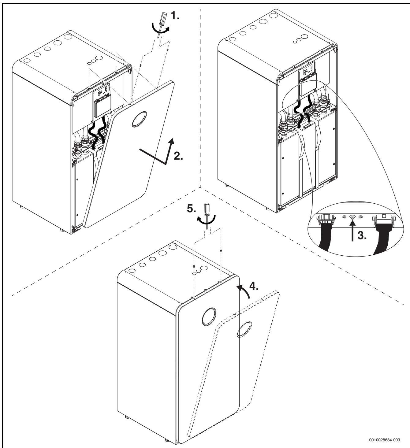
Fig. 12 Tilbakestilling av overopphetingsvern
