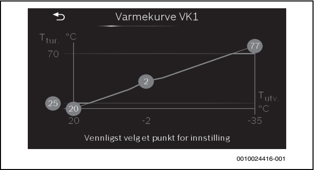
Fig. 6 Varmekurve standardvisning
