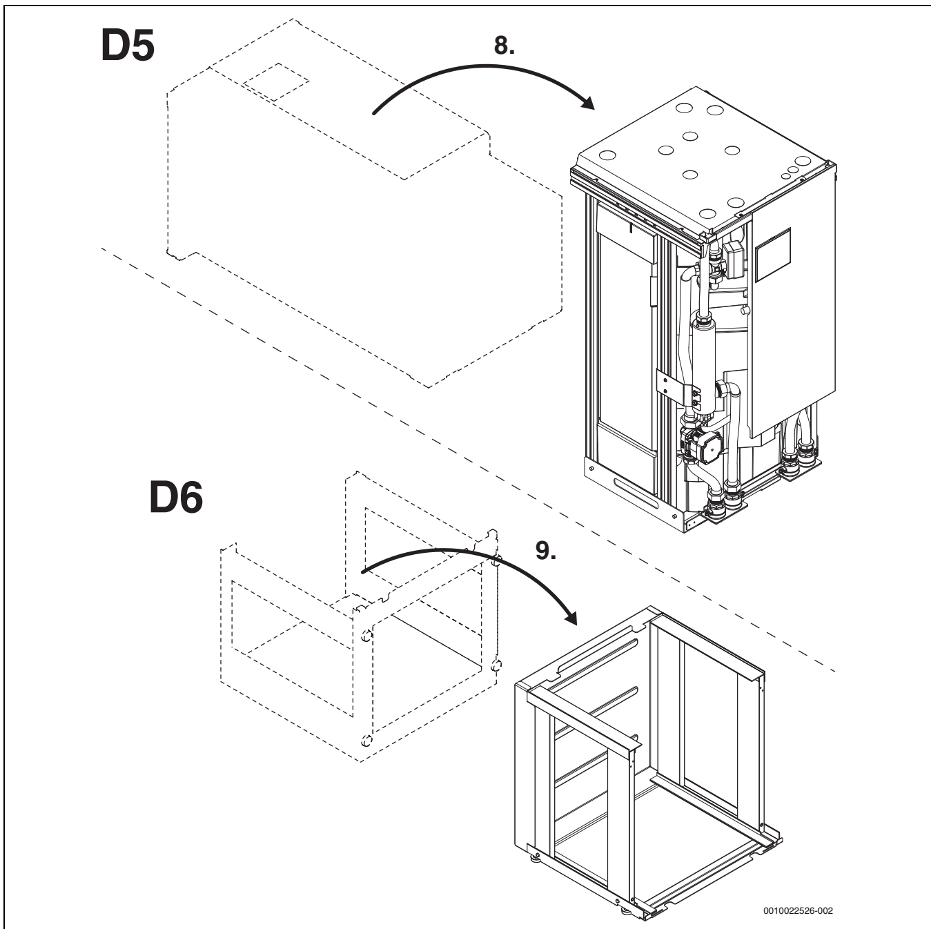
Fig. 13 Dele opp varmepumpe
