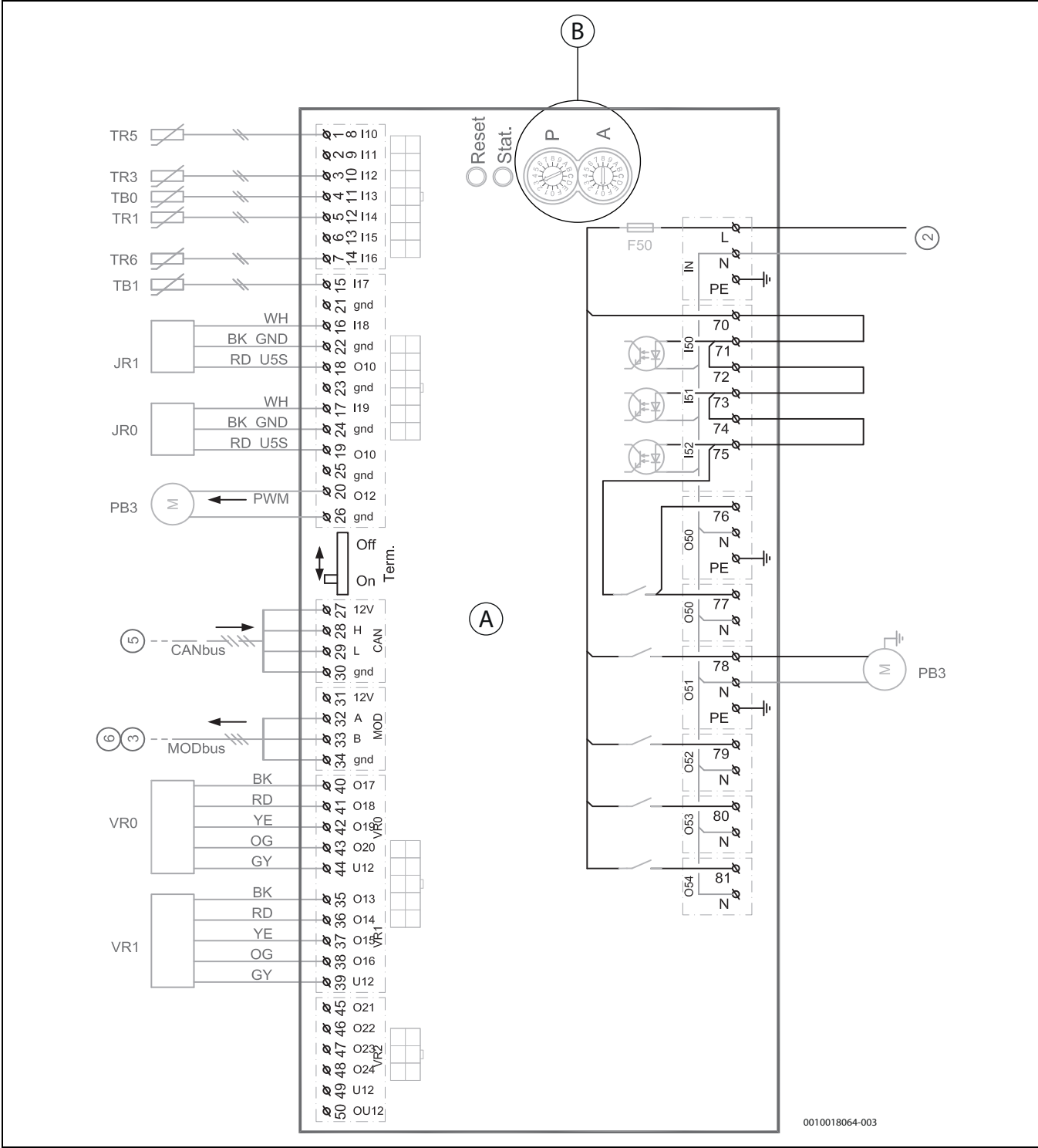
Fig. 51 Koblingsskjema I/O-modul
