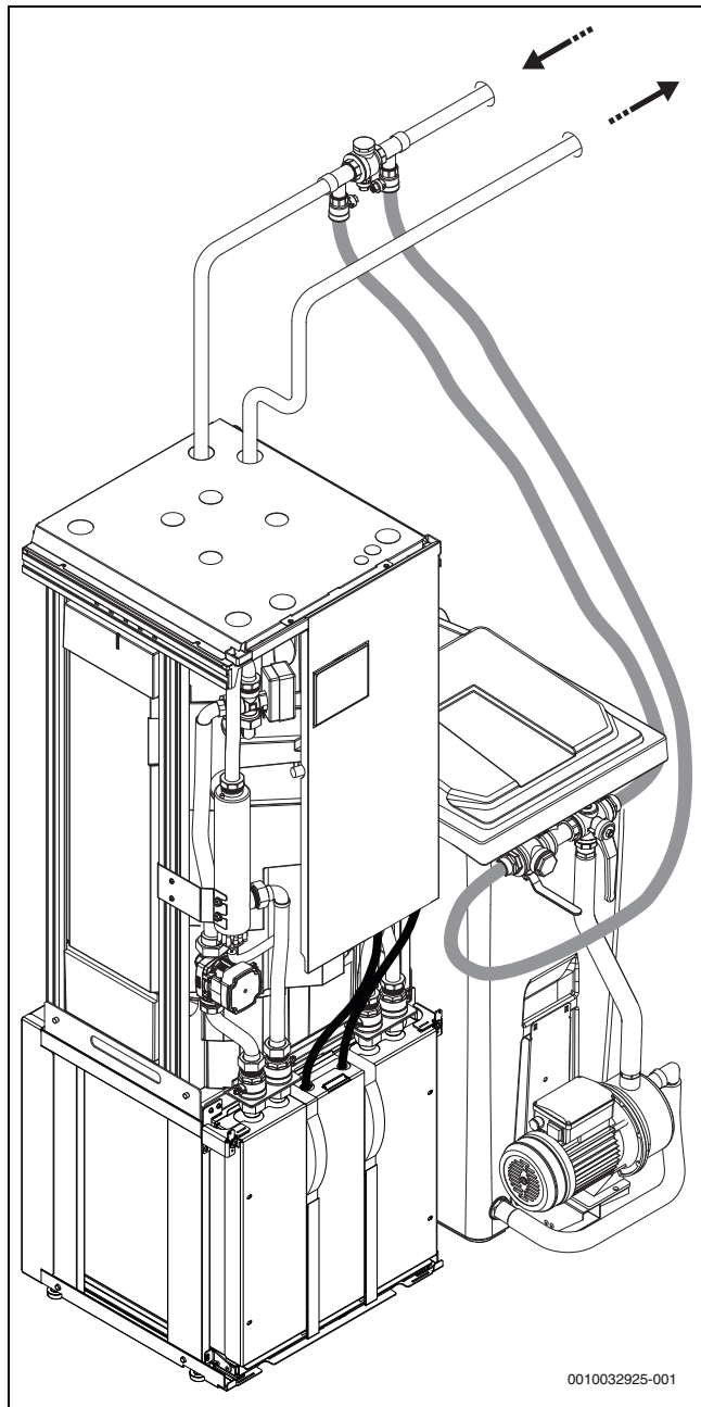
Fig. 28 Påfylling med påfyllingsstasjon
