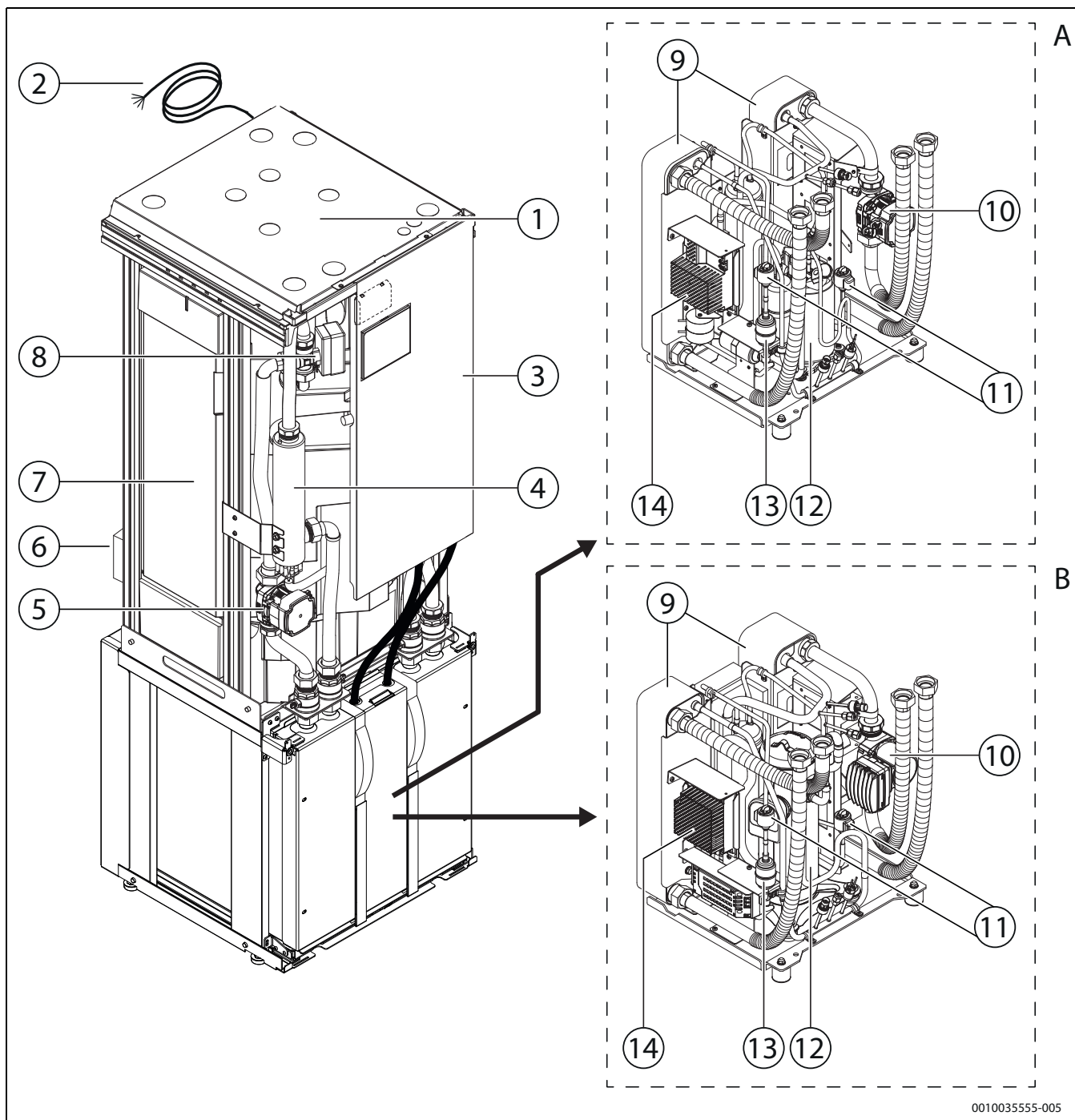
Fig. 3 Produktoversikt
