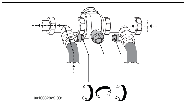
Fig. 32 Påfyllingsinnretning i trykkøkingsposisjon
