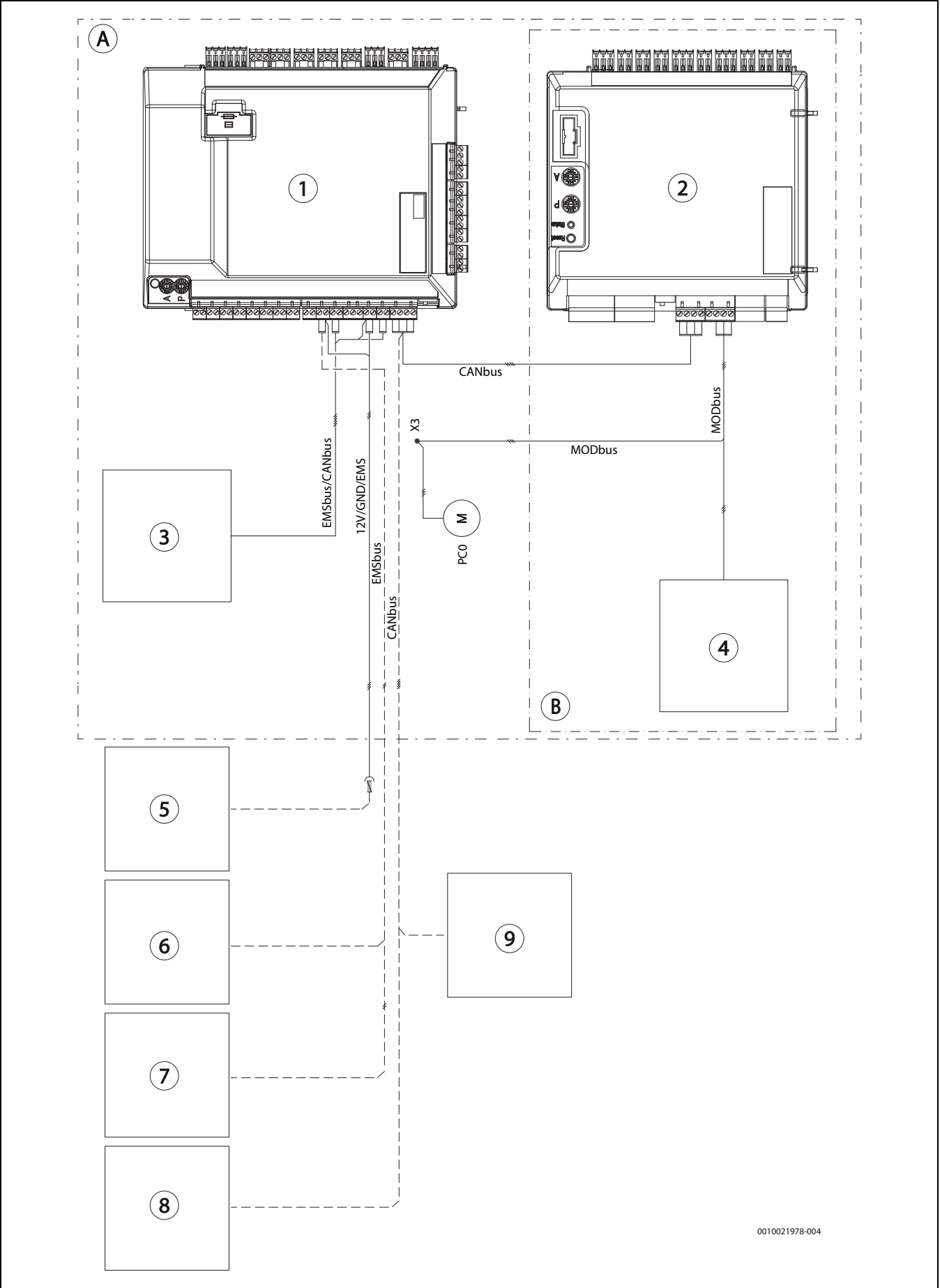
Fig. 52 Oversikt CAN-, EMS-, MOD-BUS
