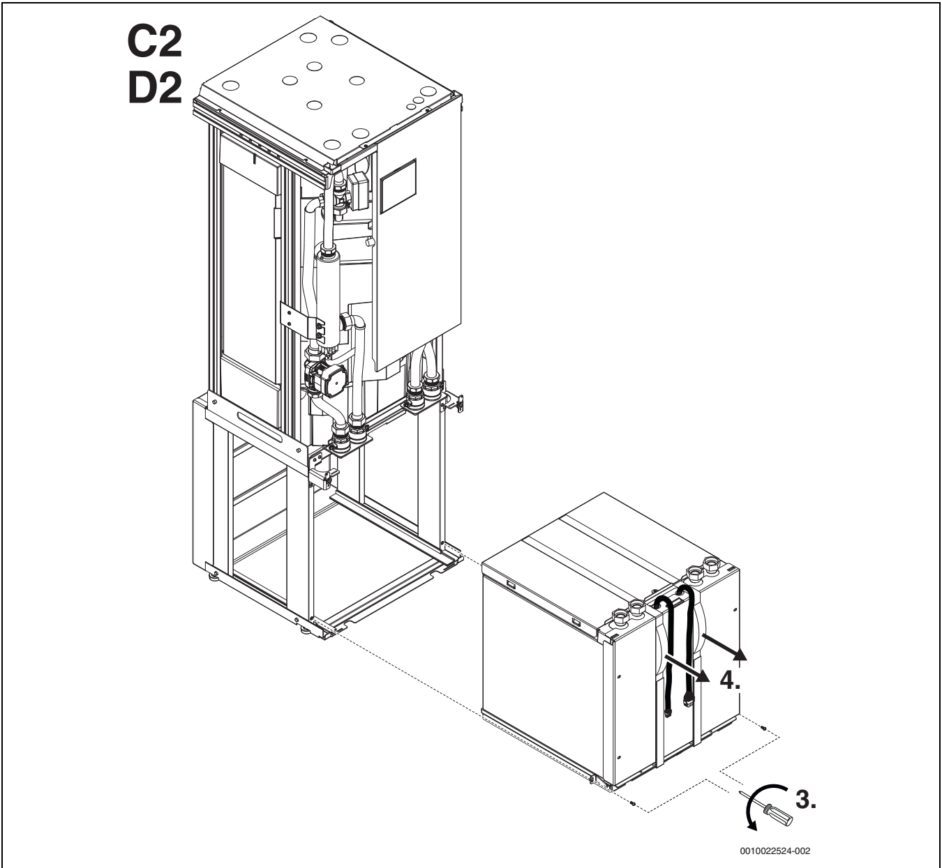
Fig. 11 Dele opp varmepumpe
