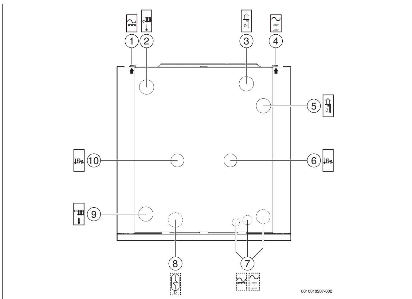
Fig. 6 Varmepumpens tilkoblinger, sett ovenfra
