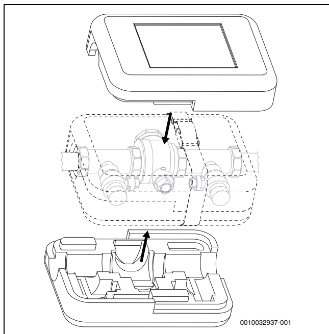
Fig. 34 Isolasjon av påfyllingsinnretningen
