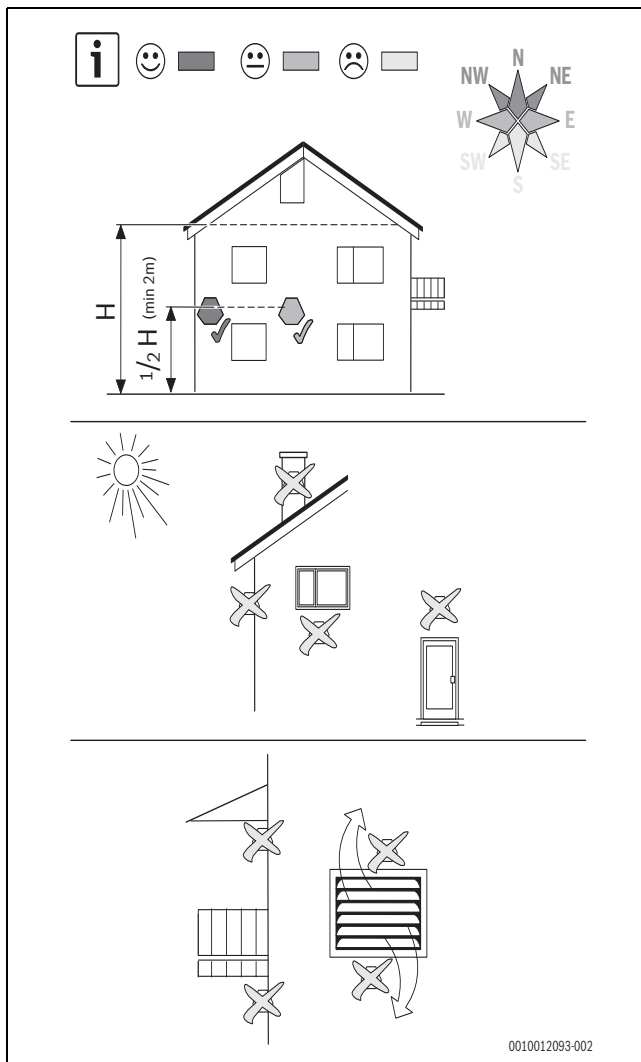
Fig. 19 Posisjonering av utetemperaturføler
