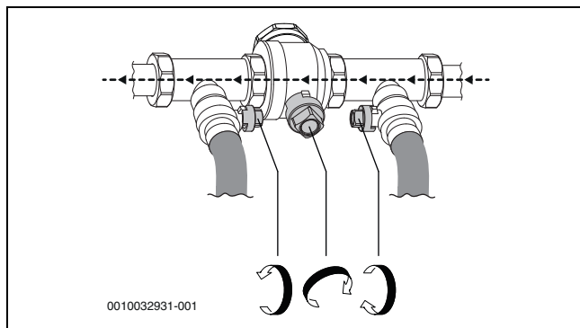
Fig. 33 Påfyllingsinnretning i normalposisjon
