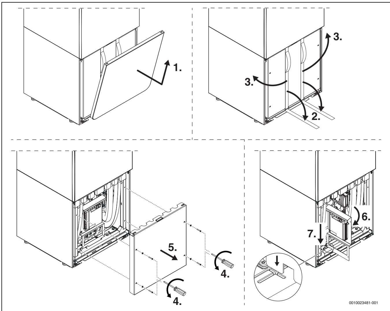
Fig. 37 Tilgang til kjølemodul ved enklere vedlikehold
