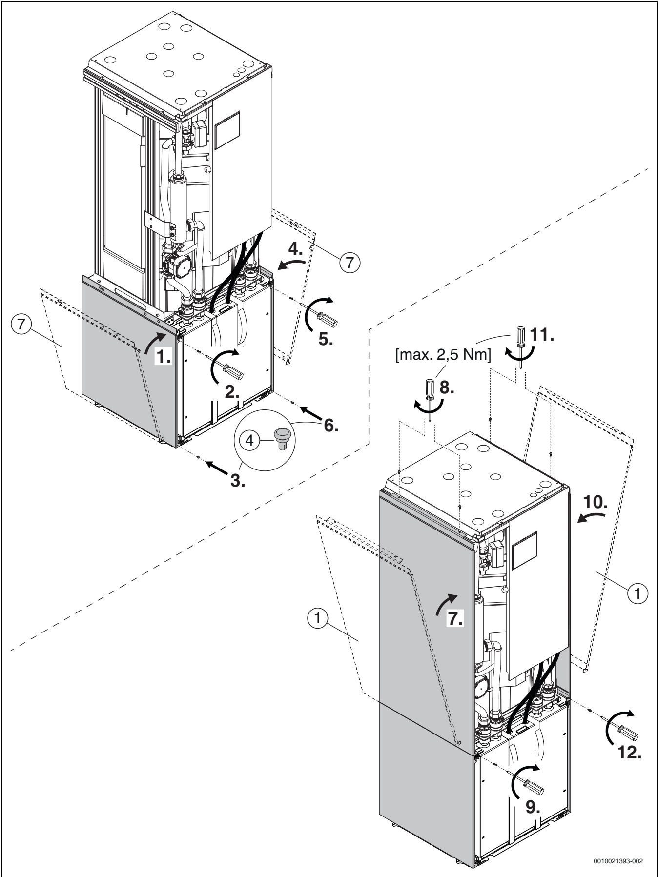
Fig. 22 Designsetmontering
