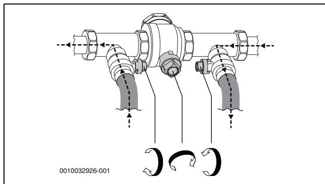
Fig. 29 Påfyllingsinnretning i påfyllingsposisjon
