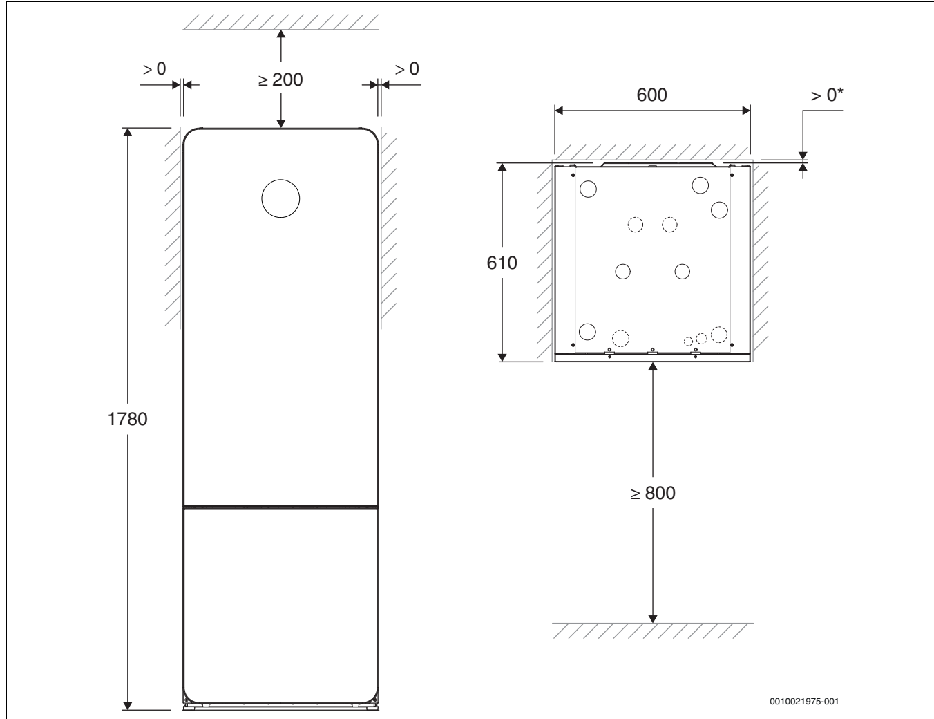
Fig. 4 Dimensjoner
