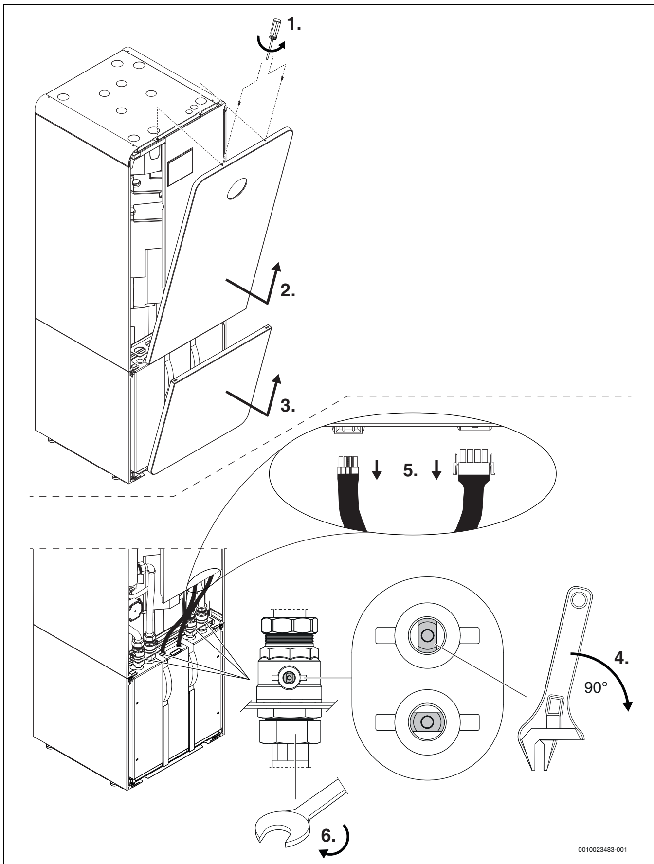
Fig. 38 Tilgang til kjølemodul ved omfattende vedlikehold, trinn 1-6
