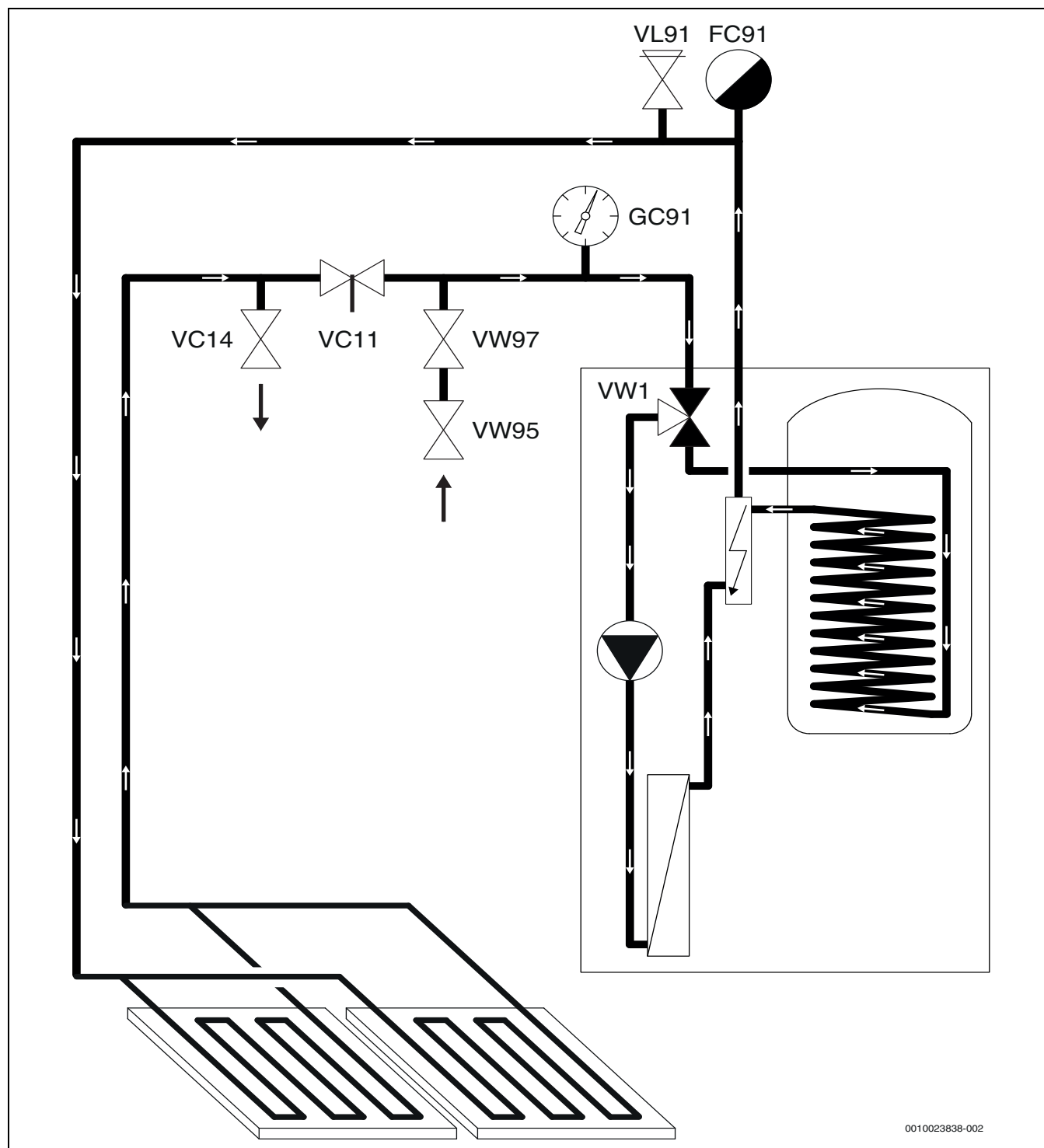
Fig. 35 Varmepumpe og varmeanlegg uten bypass
