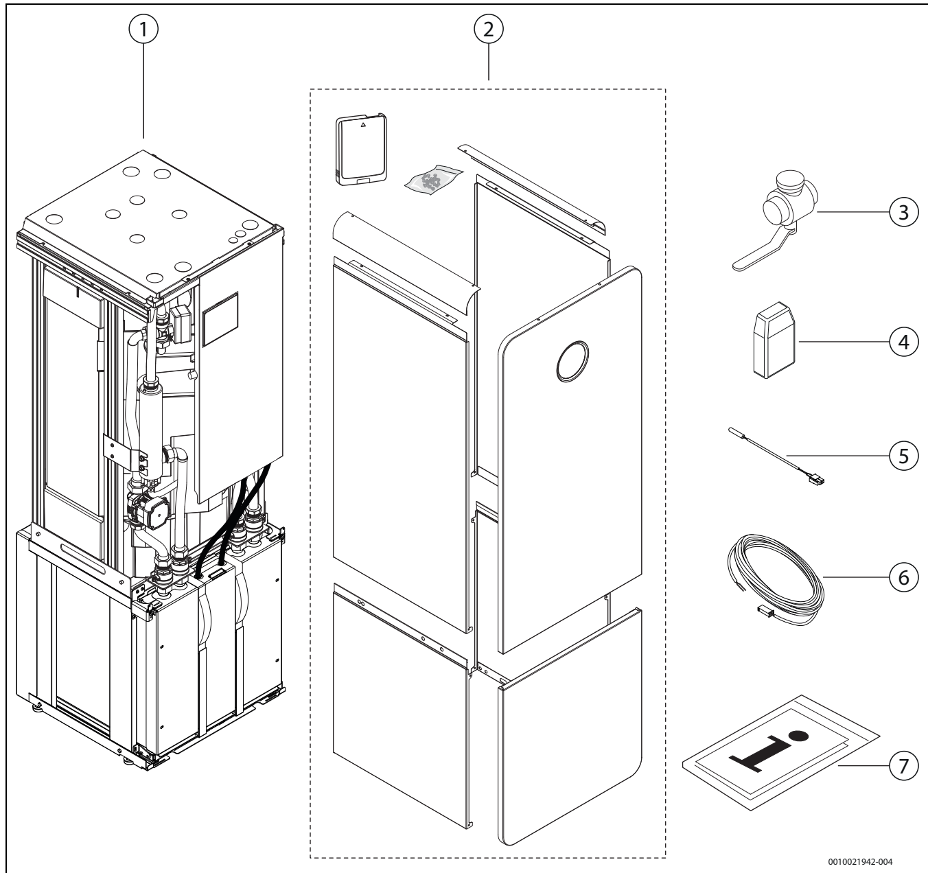
Fig. 2 Leveringsomfang
