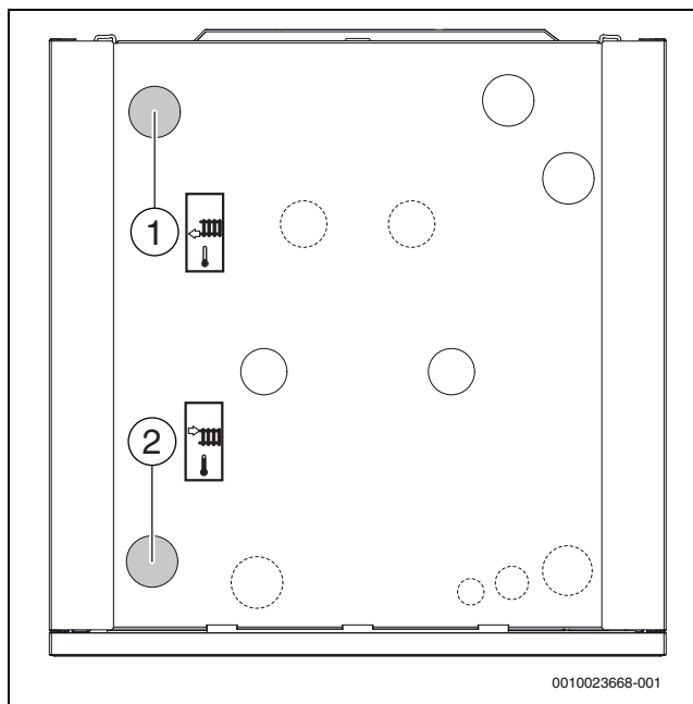
Fig. 16 Varmepumpens tilkoblinger til varmeanlegget
