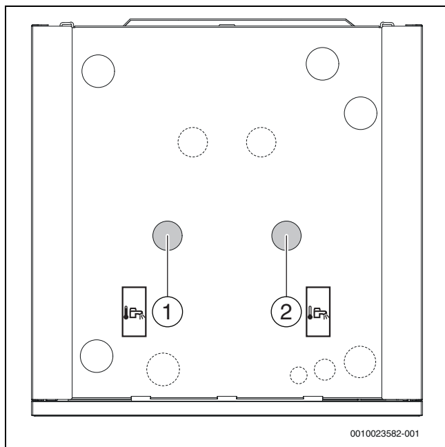
Fig. 17 Vanntilkoblinger på varmepumpen
