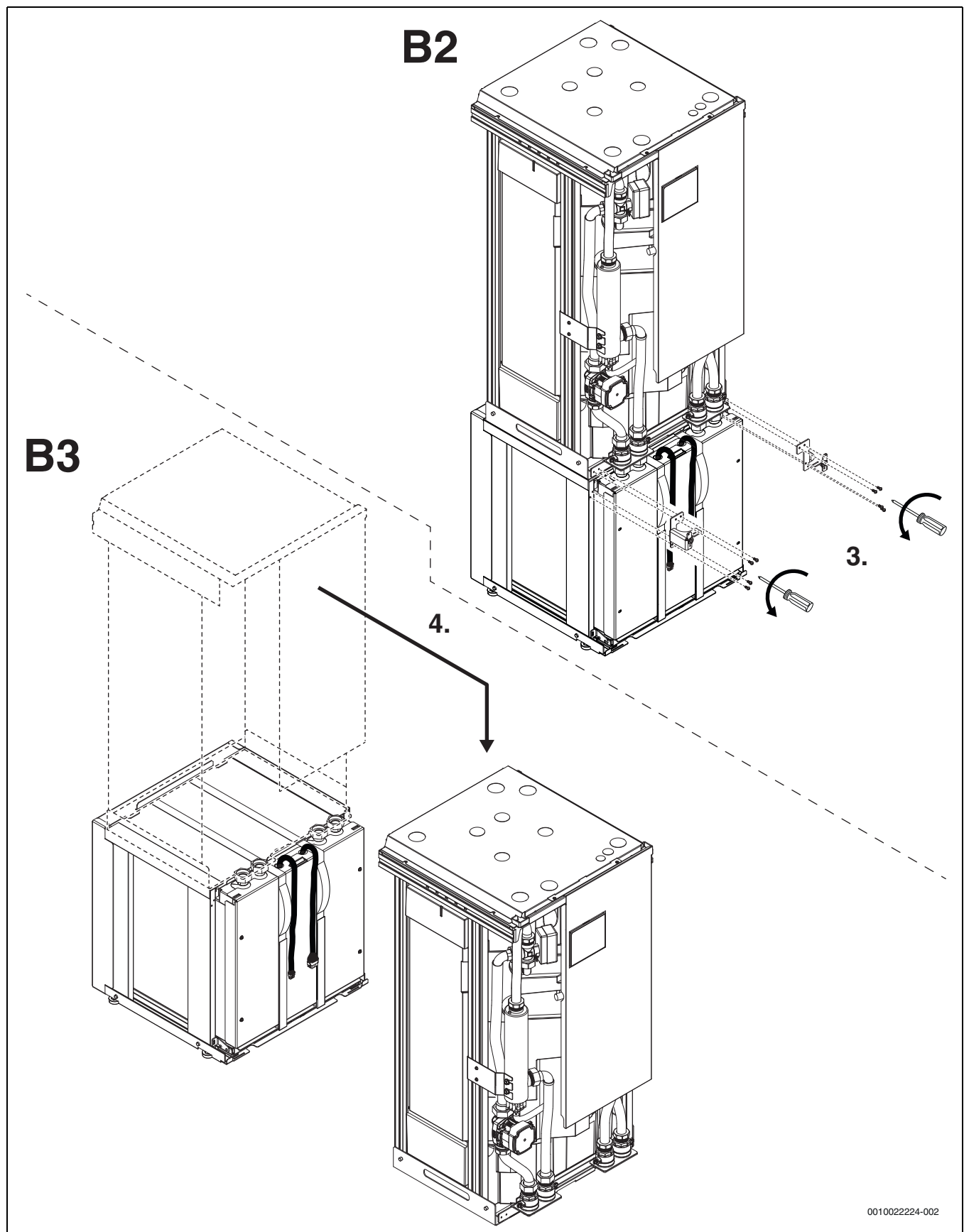
Fig. 10 Dele opp varmepumpe
