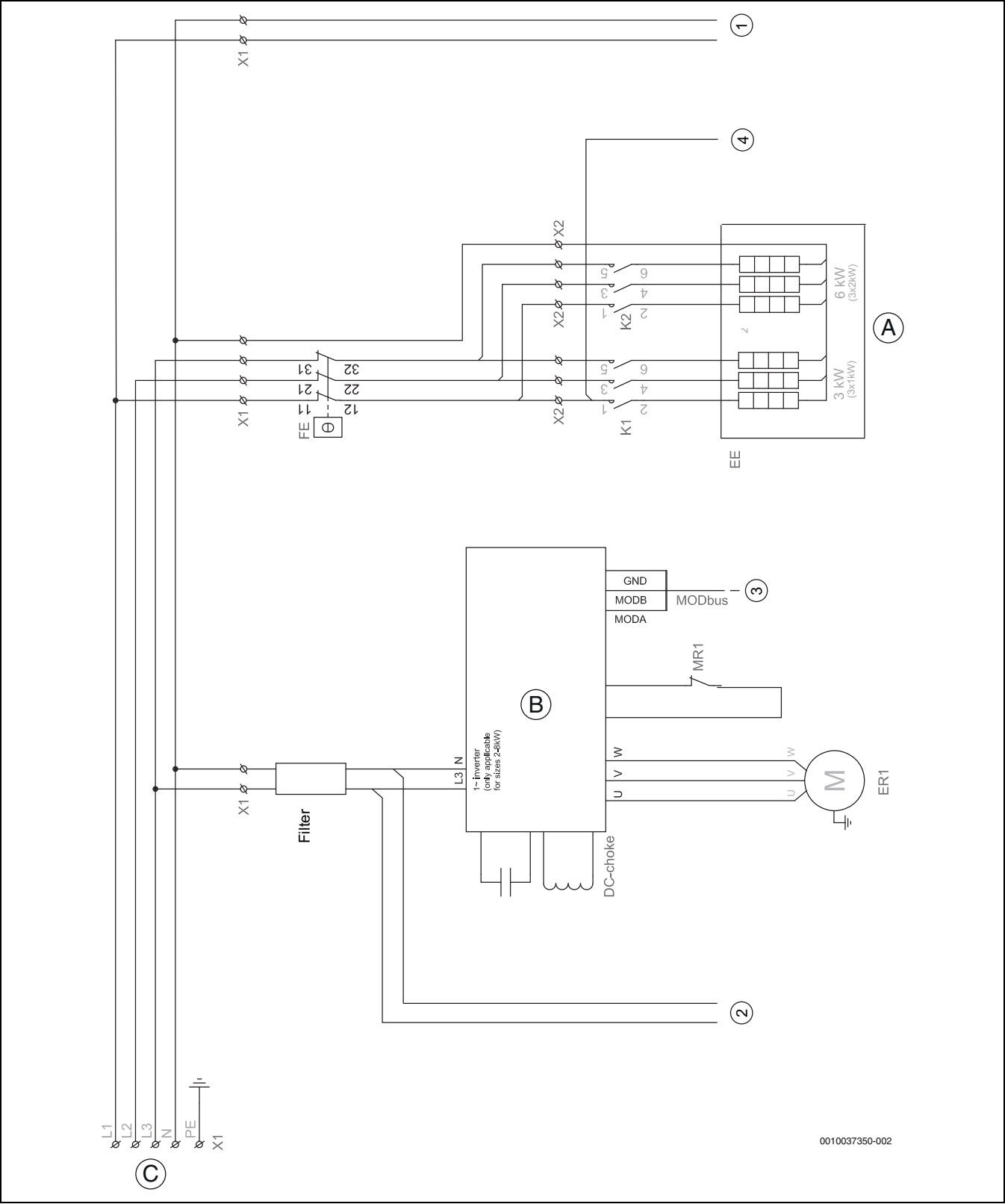
Fig. 48 Koblingsskjema hovedkrets 6–8 kW
