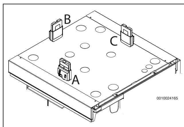
Fig. 24 Montering av holderen på det øvre varmepumpedekselet. Figuren viser holderen og Connect-Key i holderen
