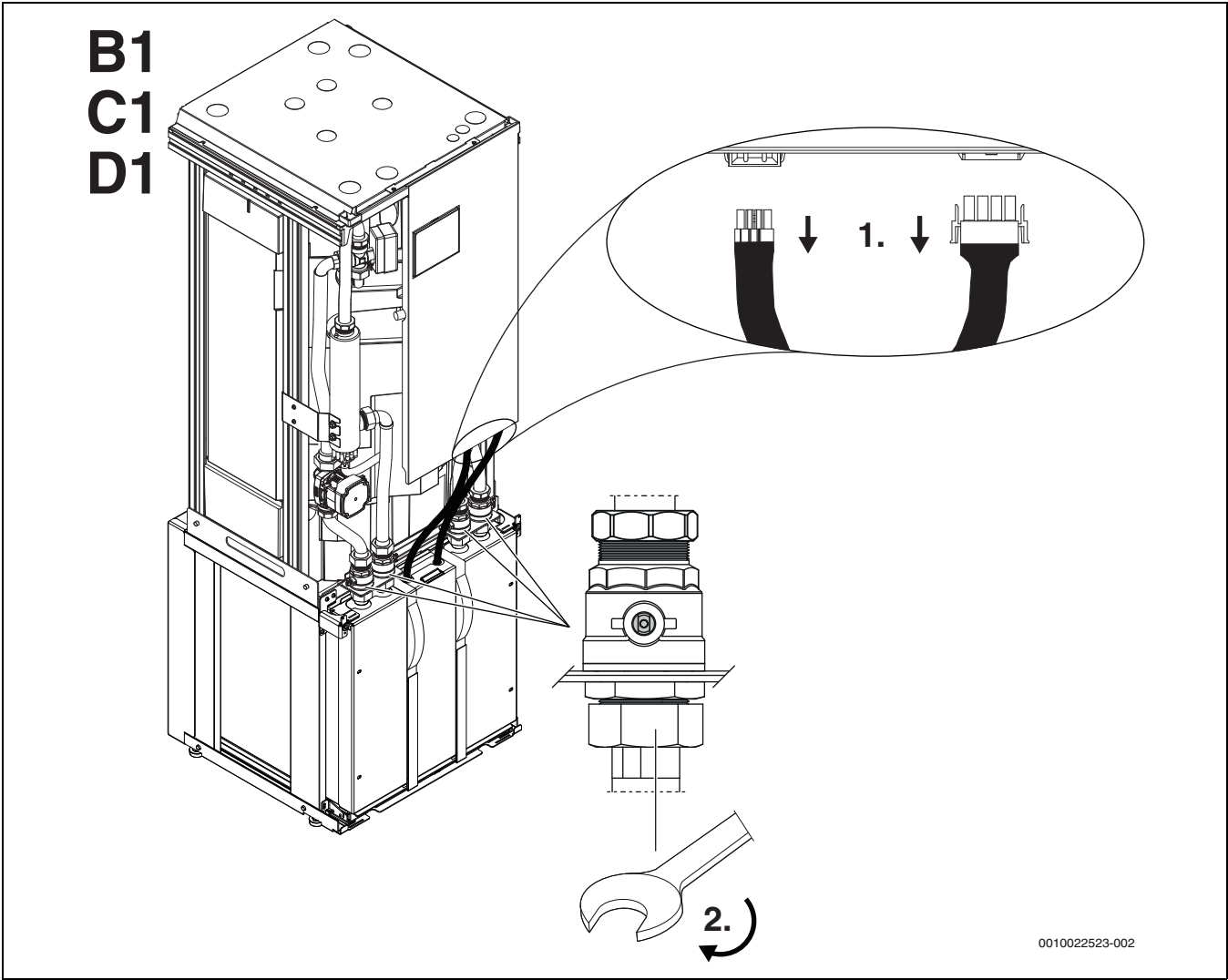
Fig. 9 Dele opp varmepumpe
