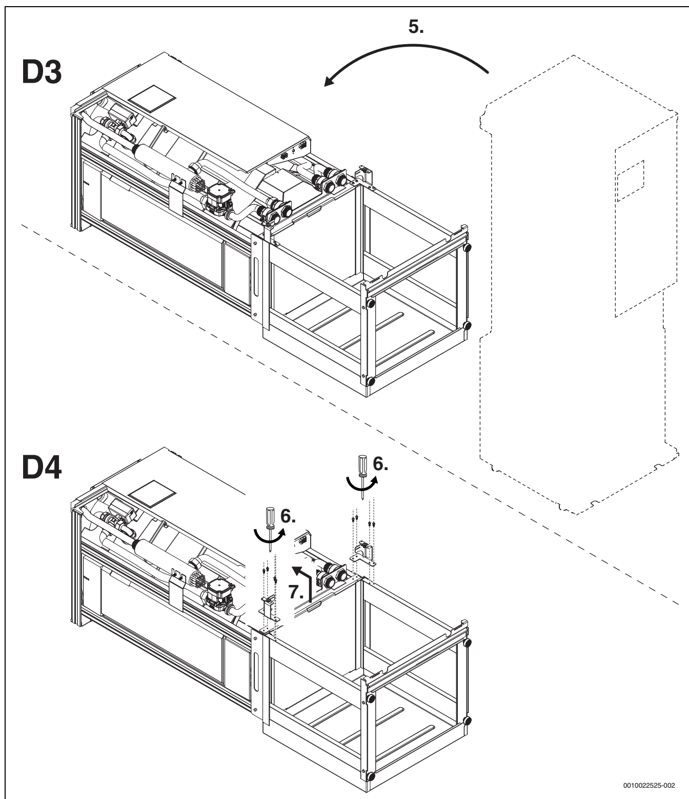
Fig. 12 Dele opp varmepumpe
