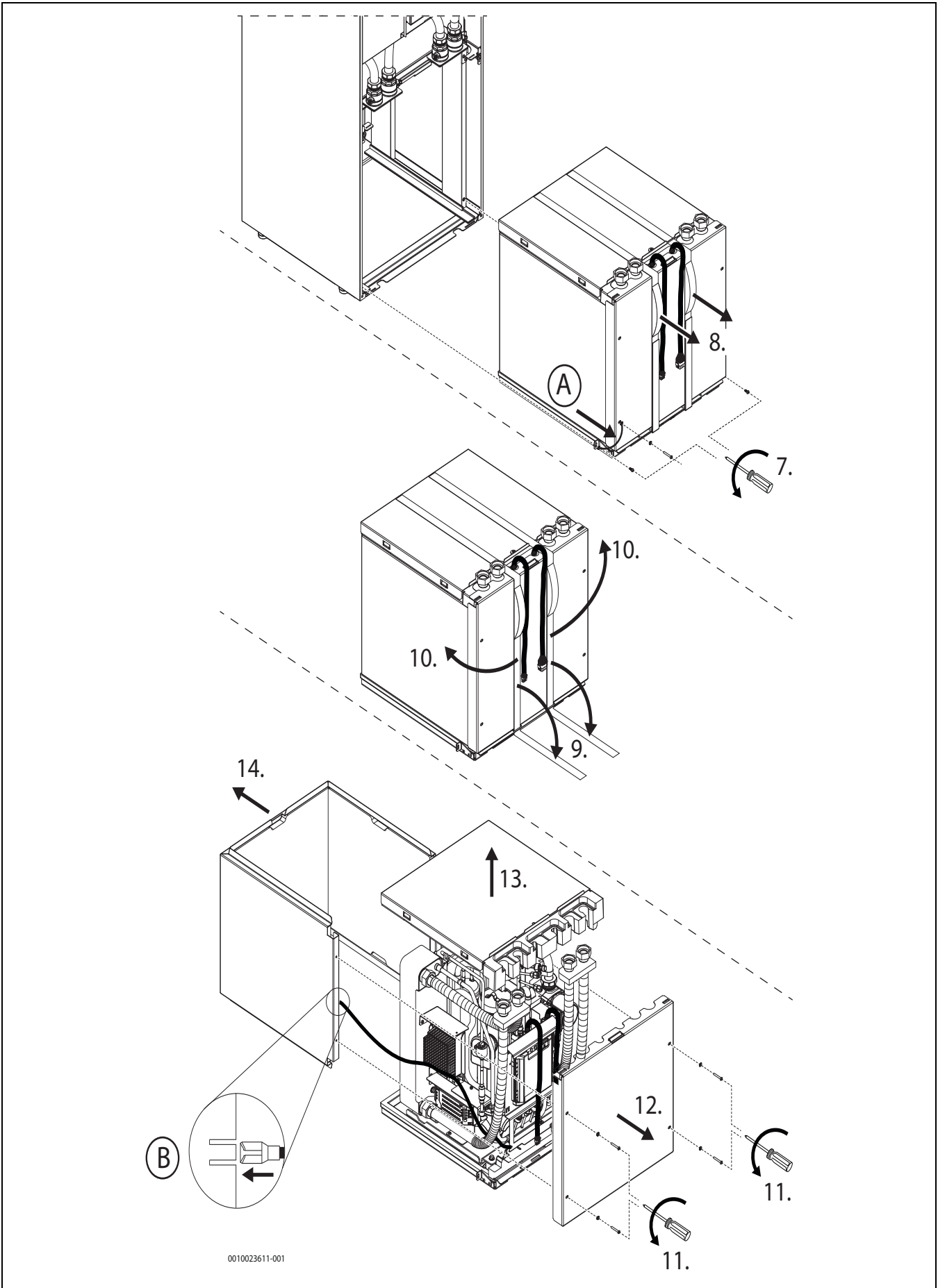
Fig. 39 Tilgang til kjølemodul ved avansert vedlikehold, trinn 7-14
