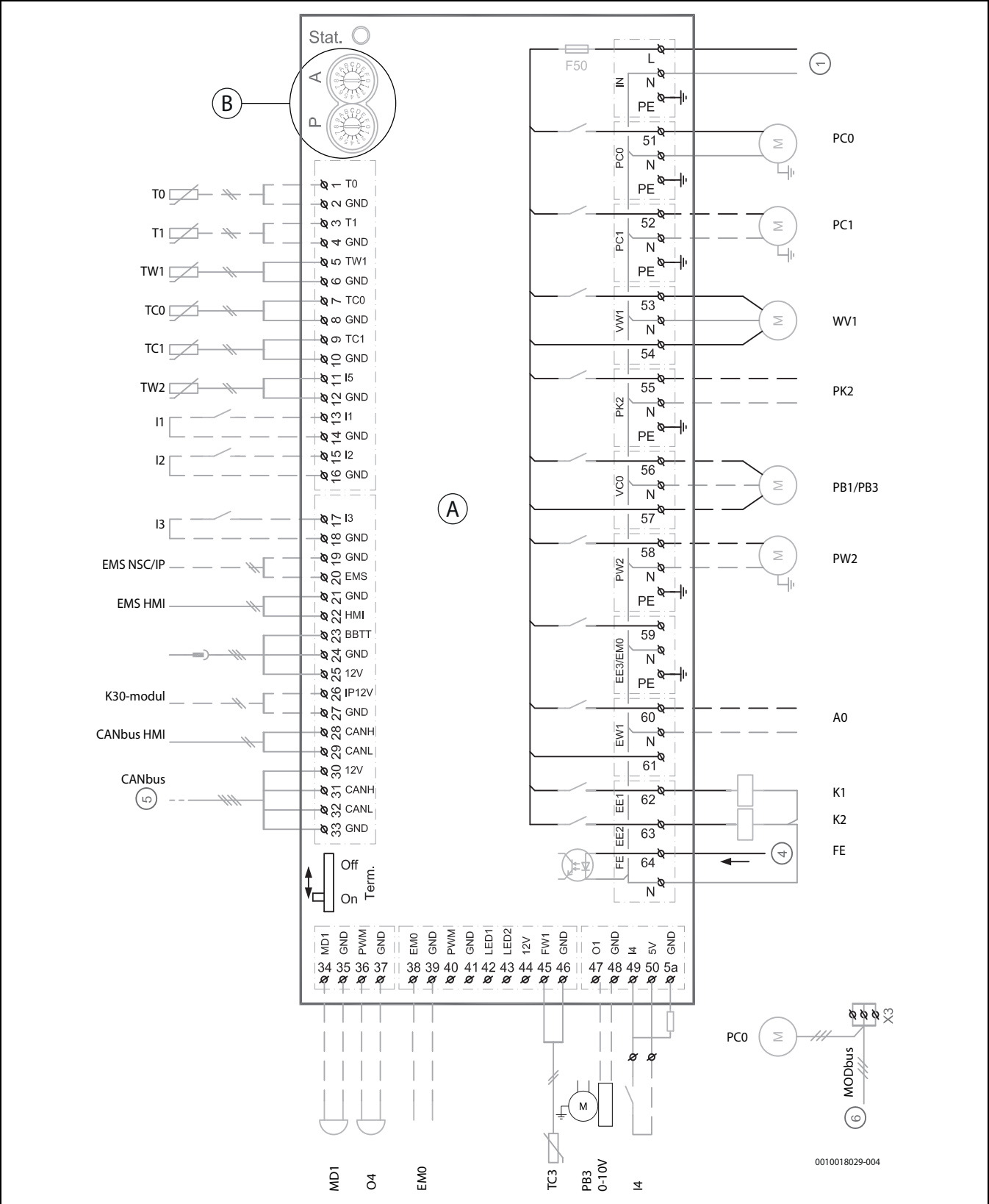
Fig. 50 Kablingsskjema installasjonskretskort
