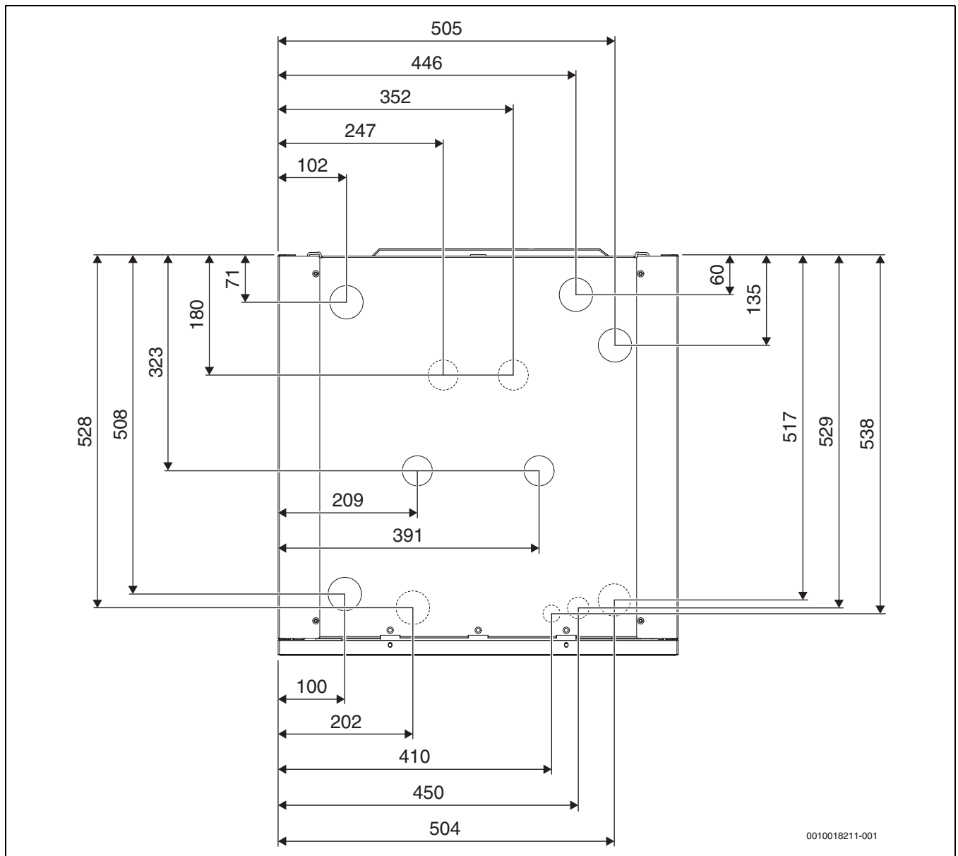
Fig. 5 Tilkoblingsdimensjoner, sett ovenfra
