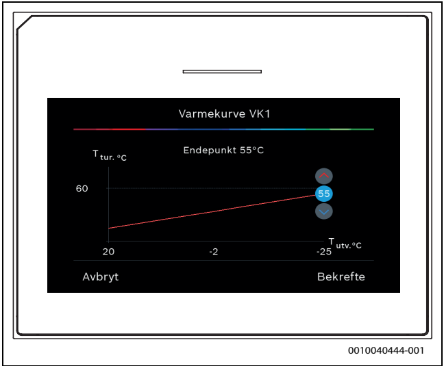
Fig. 9 Innstilling av endepunkt med et ytterligere komfortpunkt
