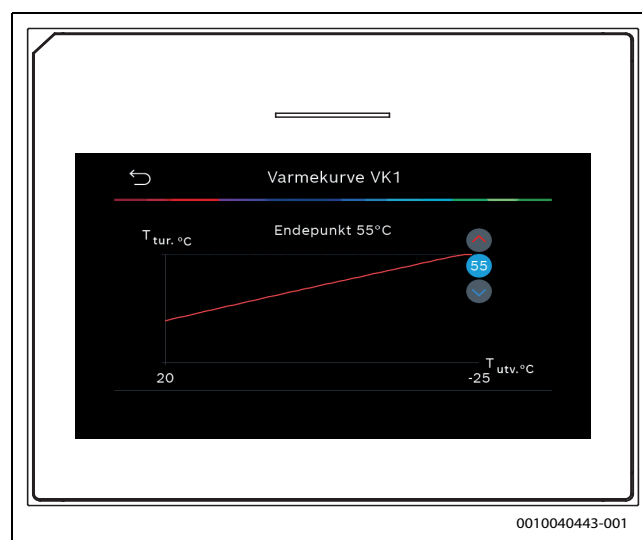
Fig. 13 Innstilling av endepunkt ved kun endepunktregulering
