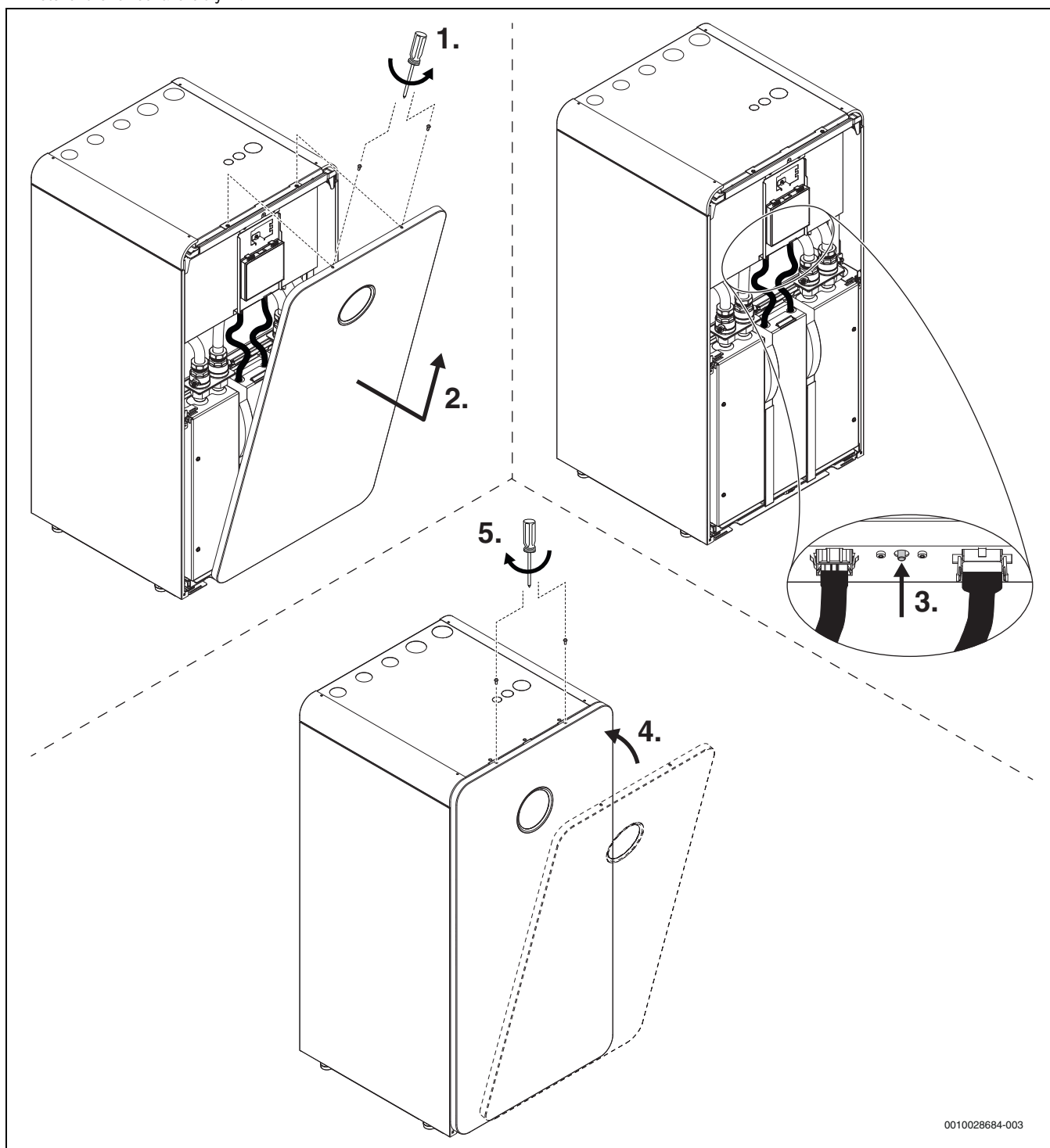
Fig. 16 Tilbakestilling av overopphetingsvern
